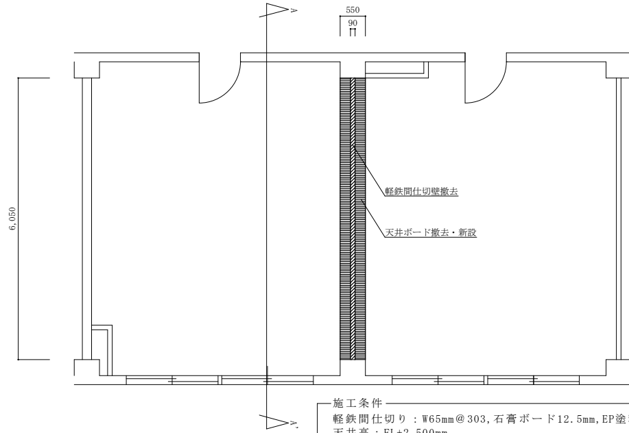
(施工前) 201号建物倉庫平面図 S=1:80
