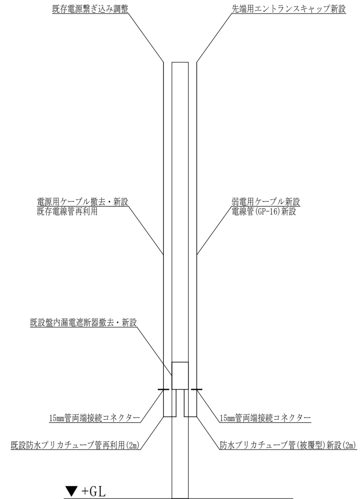
電柱①配線改修詳細図 S=1:70
