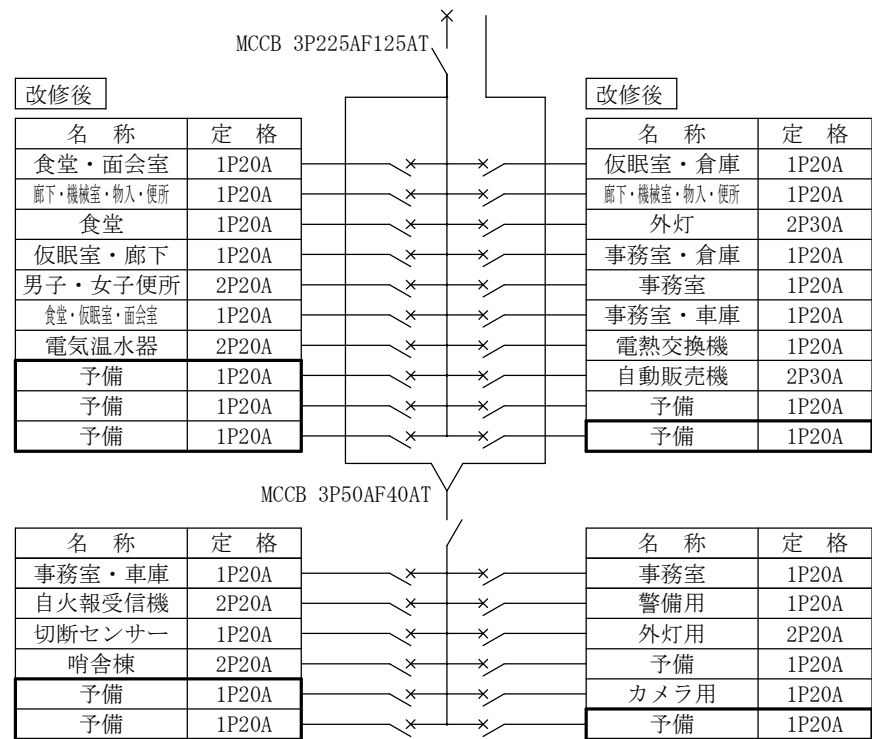
247号建物分電盤結線図（改修後）S=1：X
