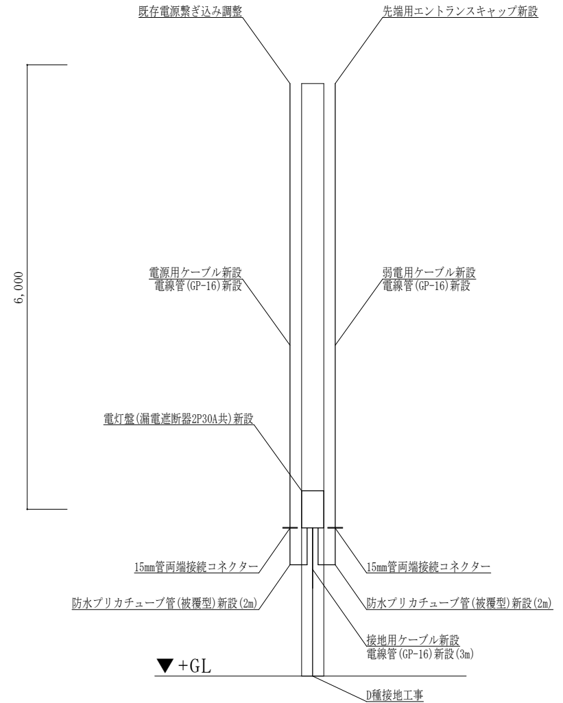
電柱②配線改修詳細図 S=1:70
