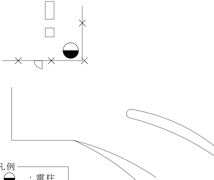
電柱②位置詳細平面図 S=1:500
