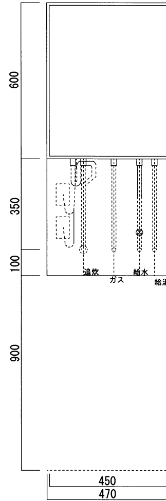
給湯器詳細図 S=1/15
