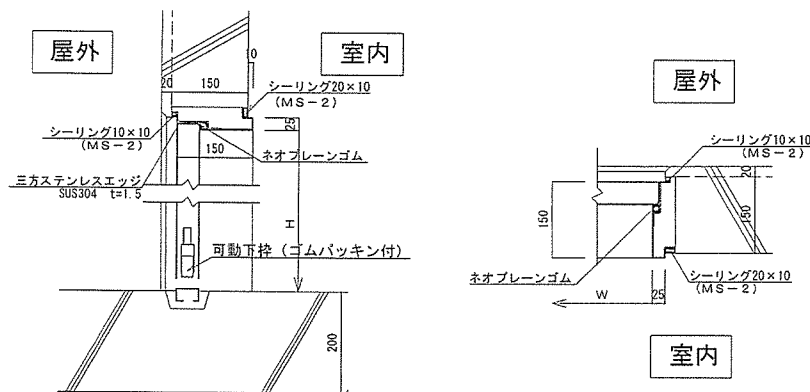
【既設】建具取付詳細図 S=1/10
