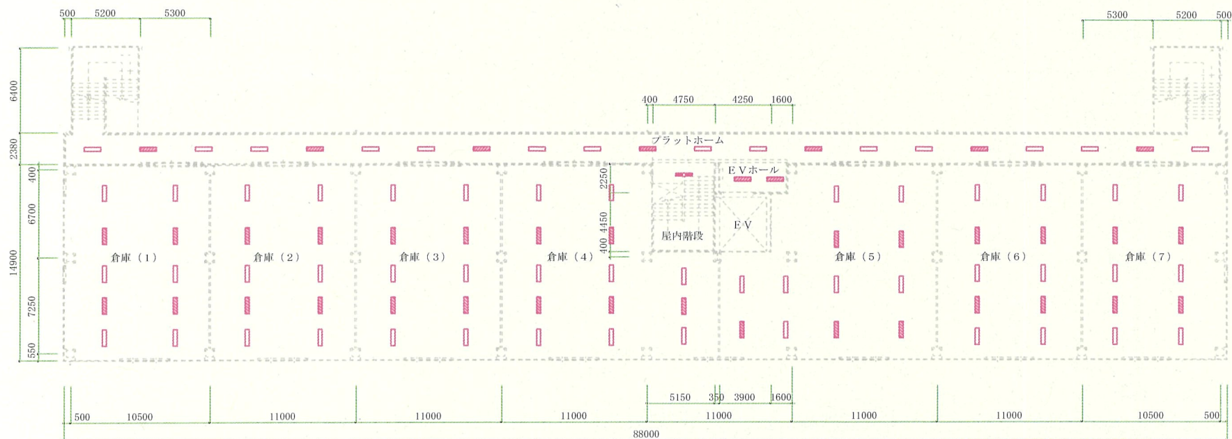
3階平面図
