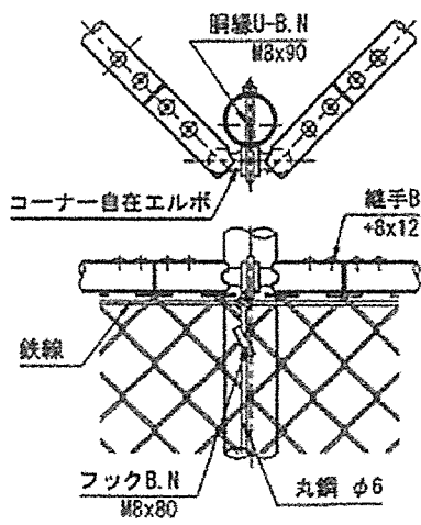
隅柱取付詳細 (コーナー自在エルボ)
