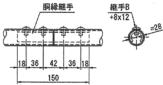
胸縁継手取付詳細
