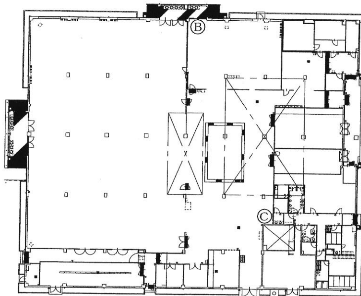
守山駐屯地97号建物平面図 S=1/450
