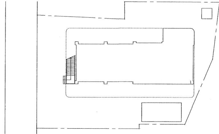
中村合同庁舎配置図 S=1/300
