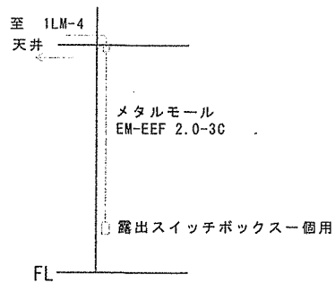
A立面図 S = 1/50
