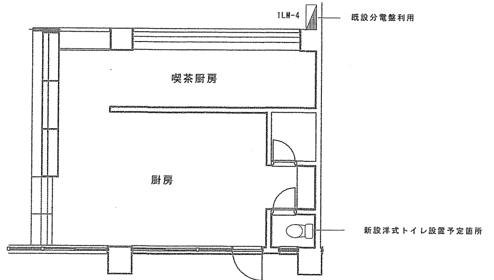
平面図 S = 1/100
