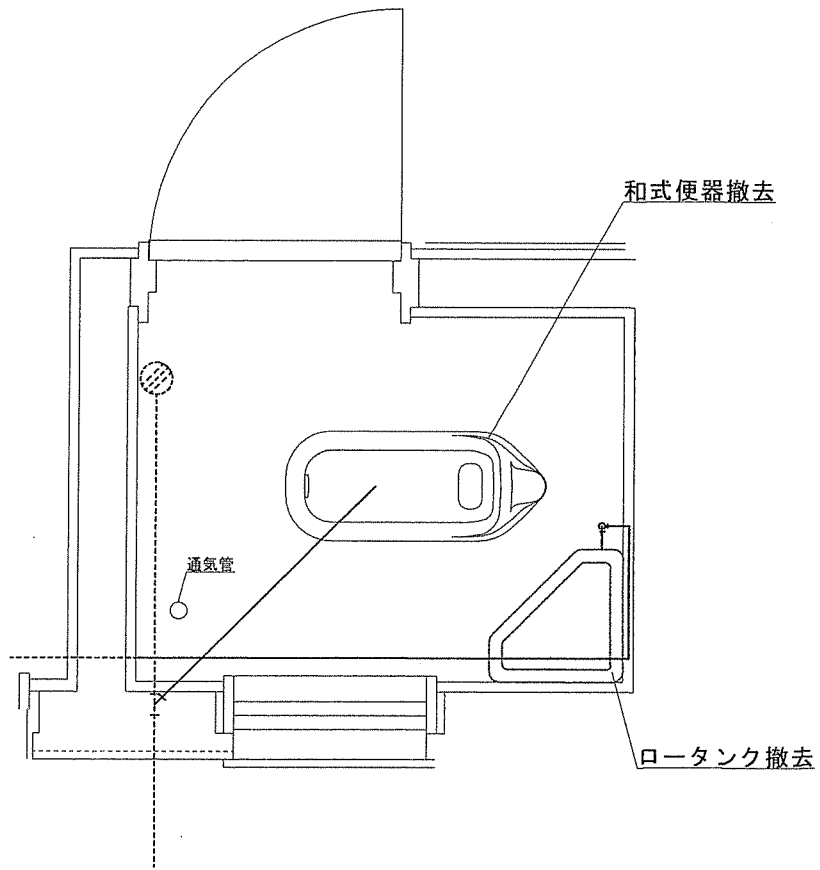
80号厚生センター1階厨房トイレ撤去平面図
