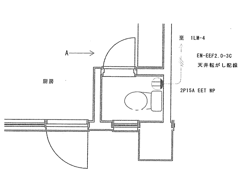
平面図 S = 1/50
