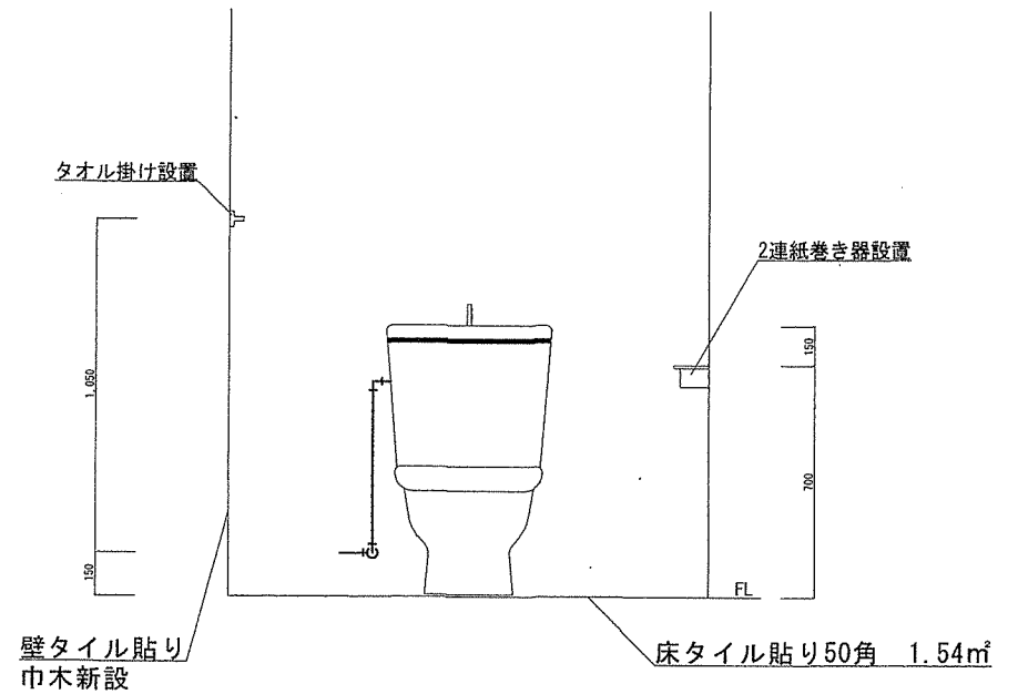
80号厚生センター1階厨房トイレ新設立面図
