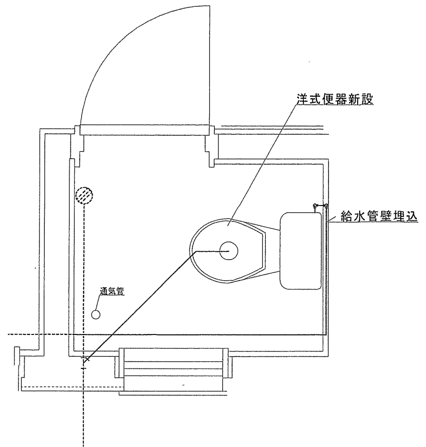
80号厚生センター1階厨房トイレ新設平面図
