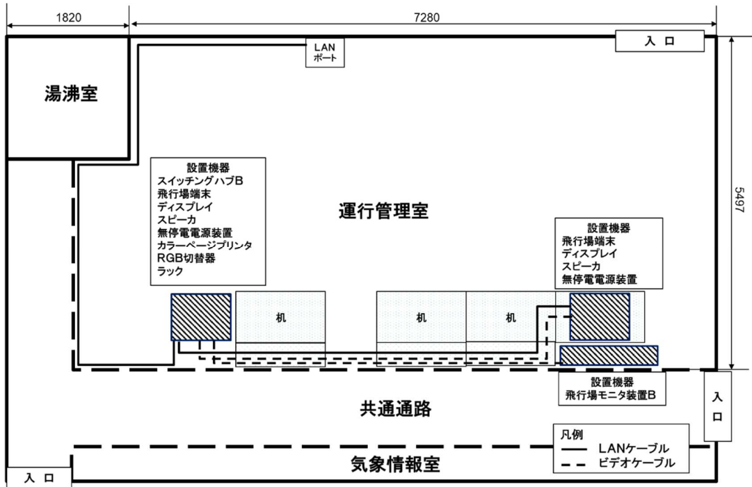
図-2 仮ベースオペレーション内配置・配線図
