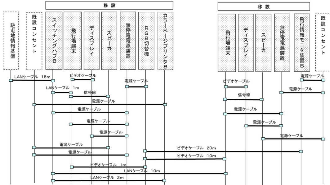
図-3 飛行管理システム配線接続図
