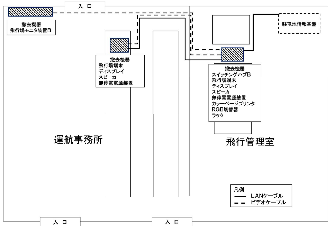
図-1 現ベースオオペレーション内配置・配線図
