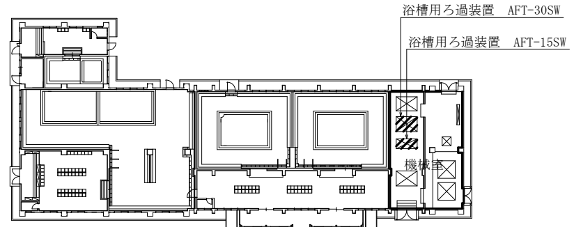
浴場平面図 S : 1 / 600
