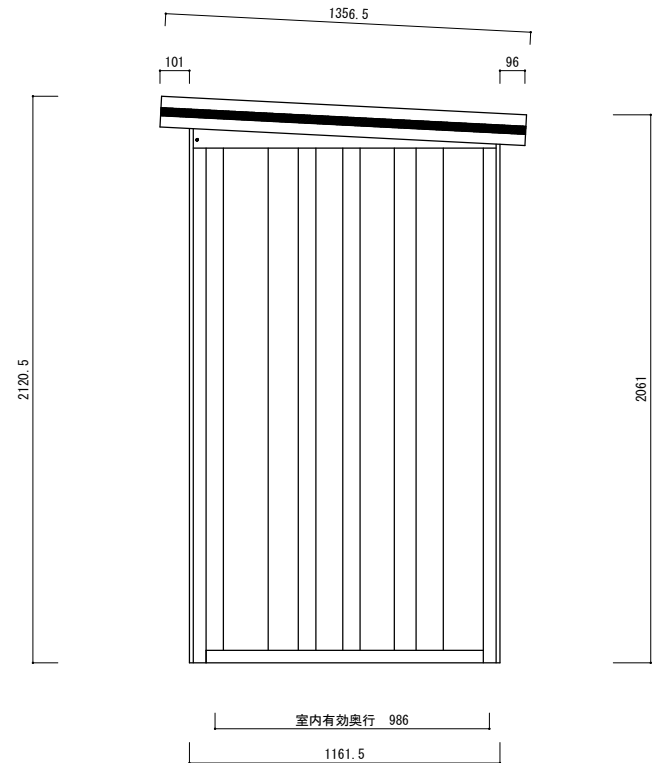
物置側面標準図
