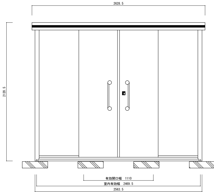
物置正面標準図
