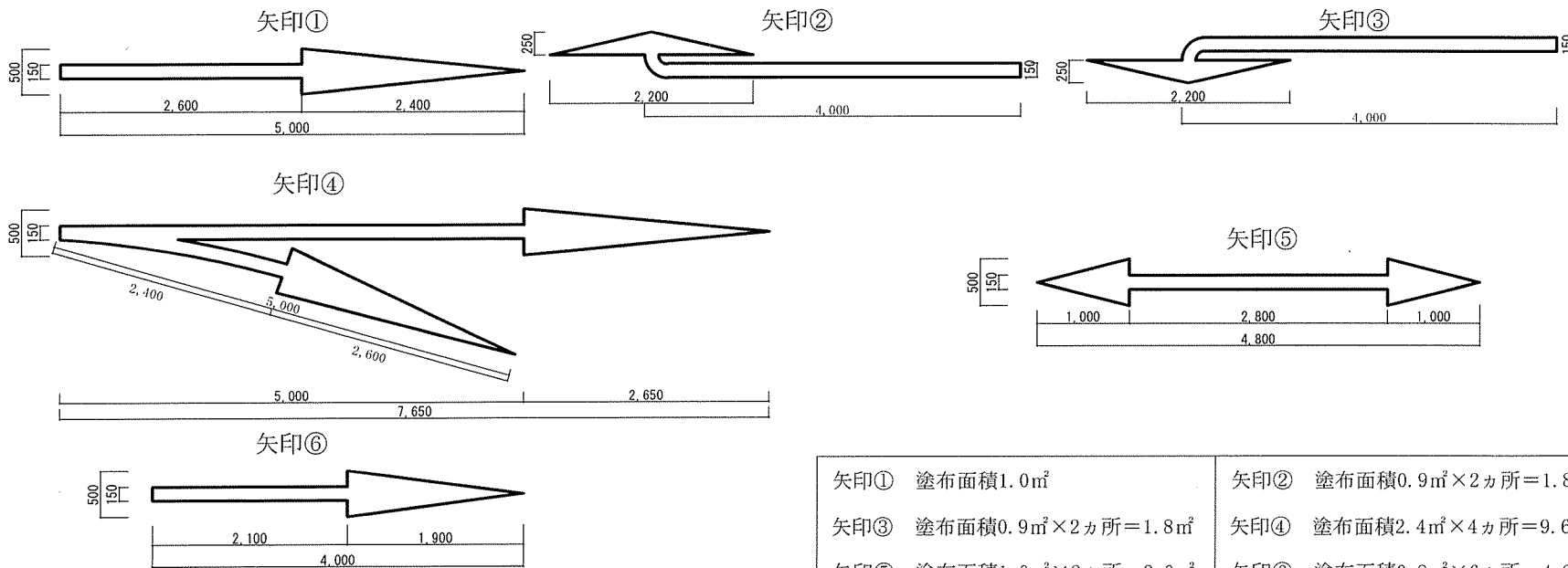
寸法表 1 / 7 5
