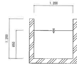
No.2 断面図 (土砂分離槽)
