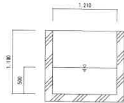
No.1 断面図 (既設洗車場)
