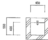
No.3 断面図 (ため柵)
