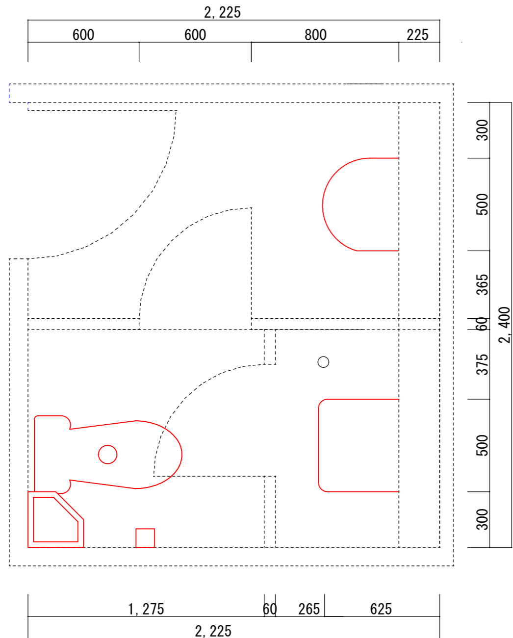
【改修前】衛生設備工事 女性トイレ平面図
