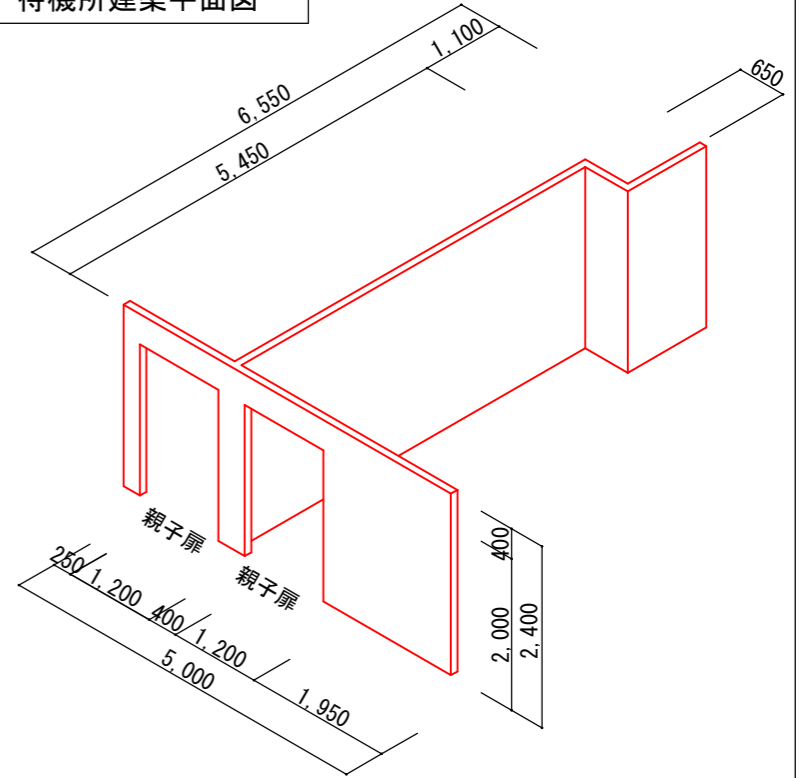
【改修後】待機所建築平面図
