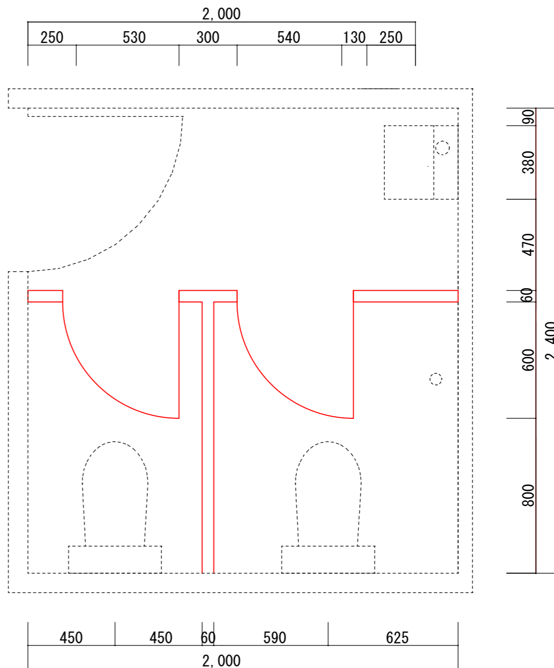
【改修後】ブース取替工事 女性トイレ平面図
