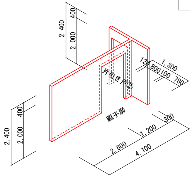
【新設】間仕切り壁 透視図
