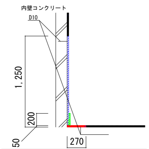
【改修後】女性トイレ内壁 断面図
