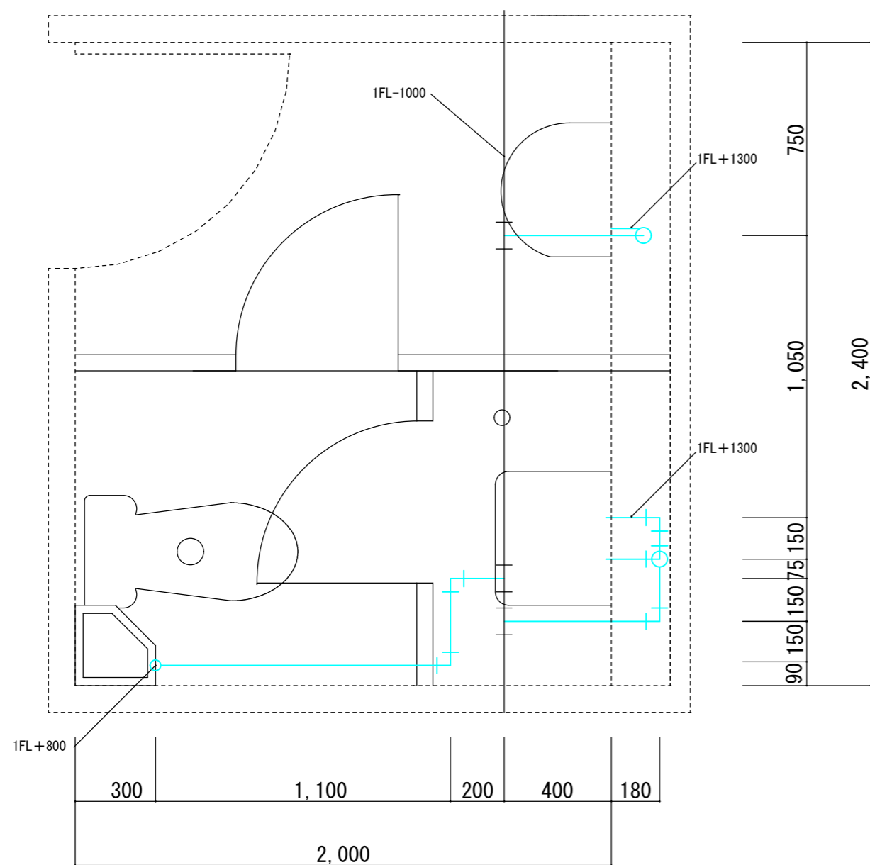
【改修前】給水管工事 女性トイレ平面図
