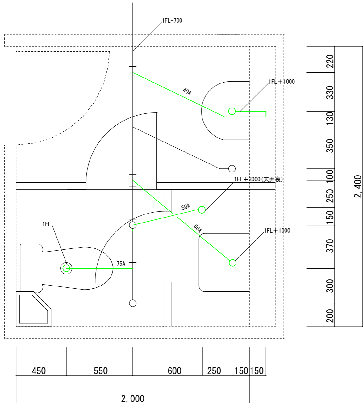
【改修前】排水管工事 女性トイレ平面図
