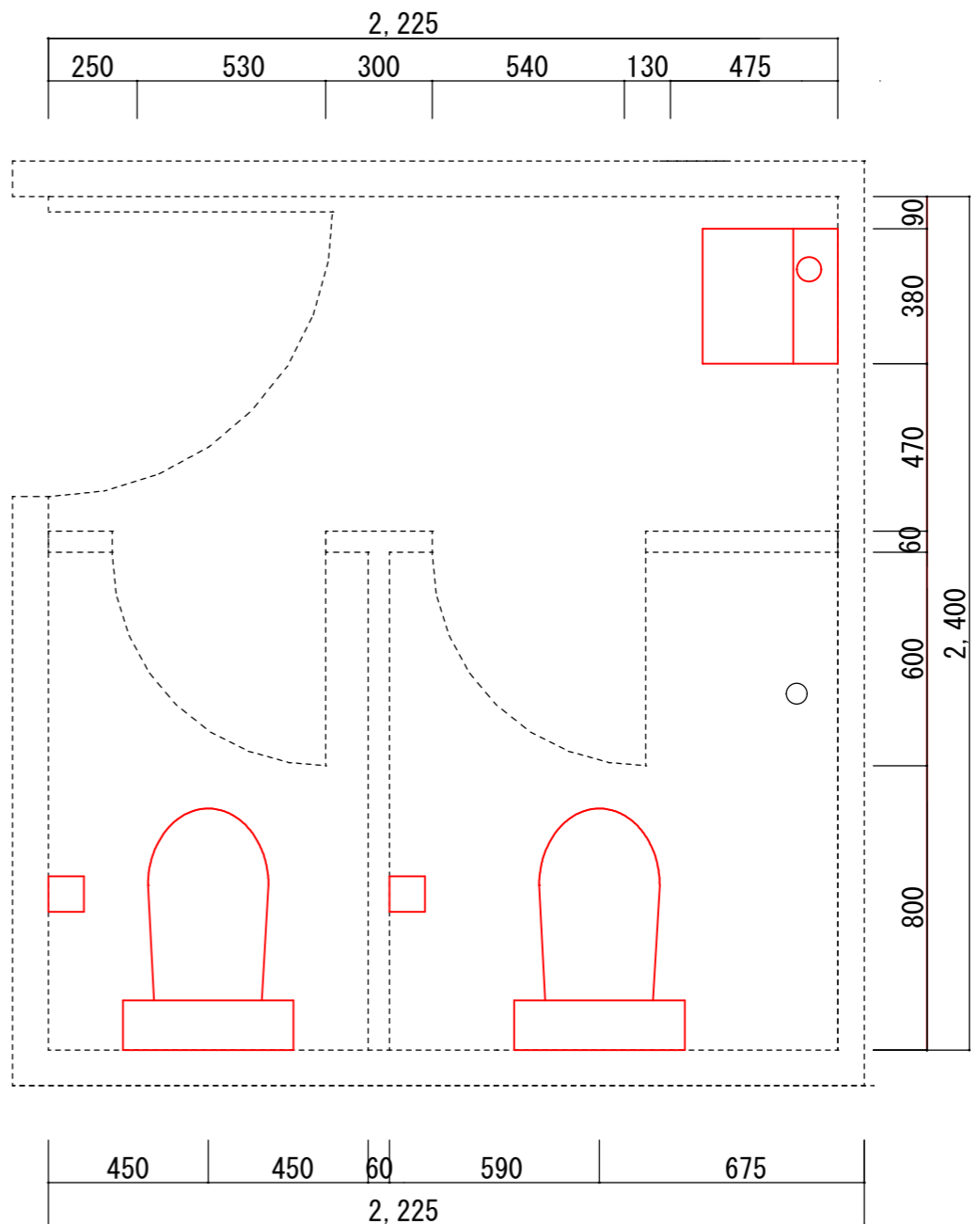
【改修後】衛生設備工事 女性トイレ平面図
