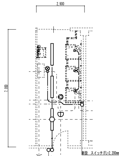
電気設備図 改修図 S=1/100
