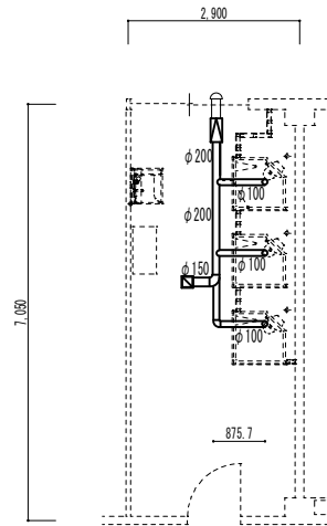
換気設備図 改修図 S=1/100
