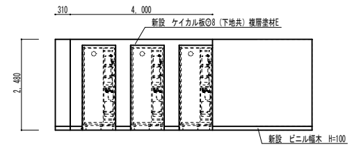
展開図 改修図 S=1/100
