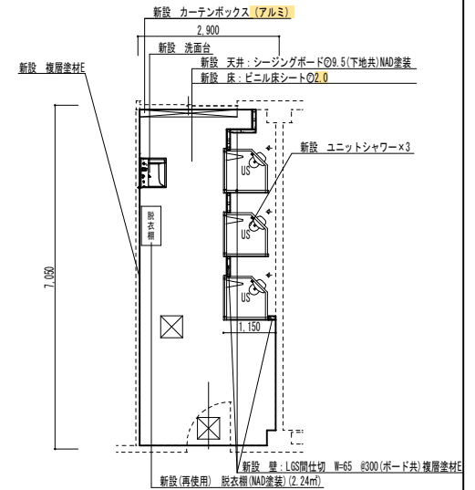
平面詳細図 改修図 S=1/100
