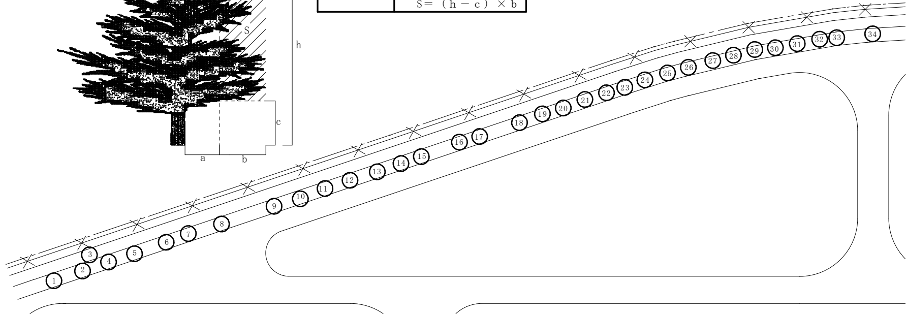
配置図 S = 1 / X
