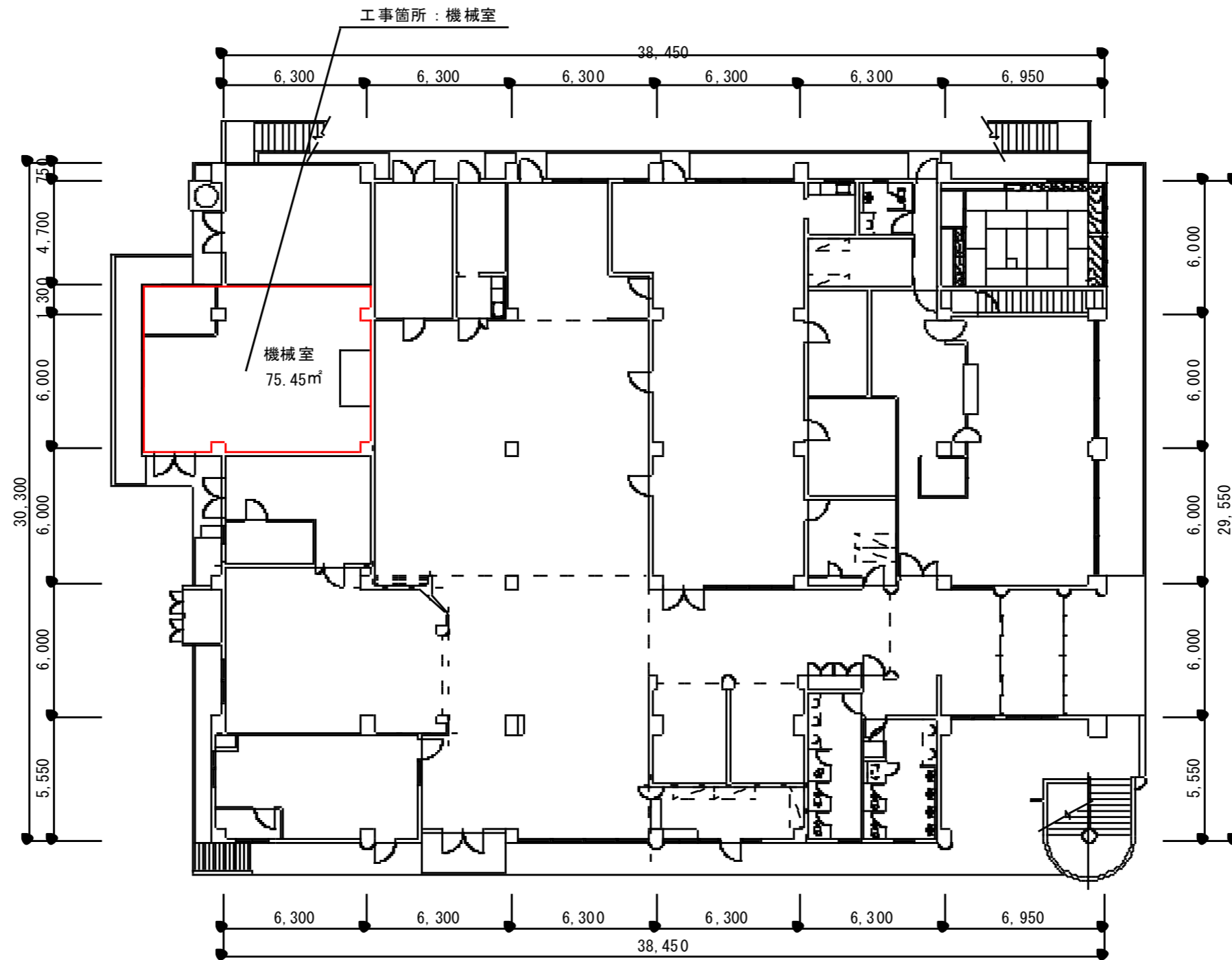
112号建物1階平面図 S=1/300
