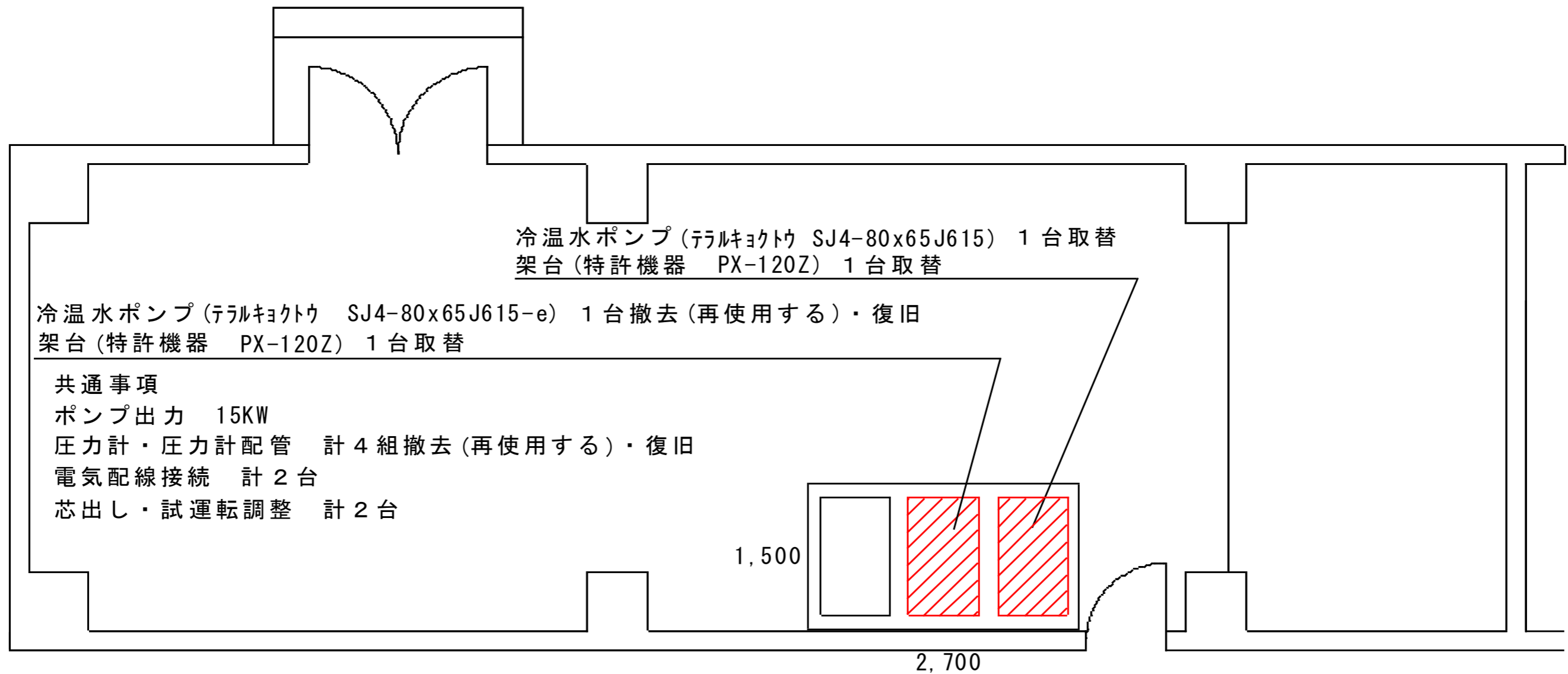
109号建物機械室平面図 S=1/60
