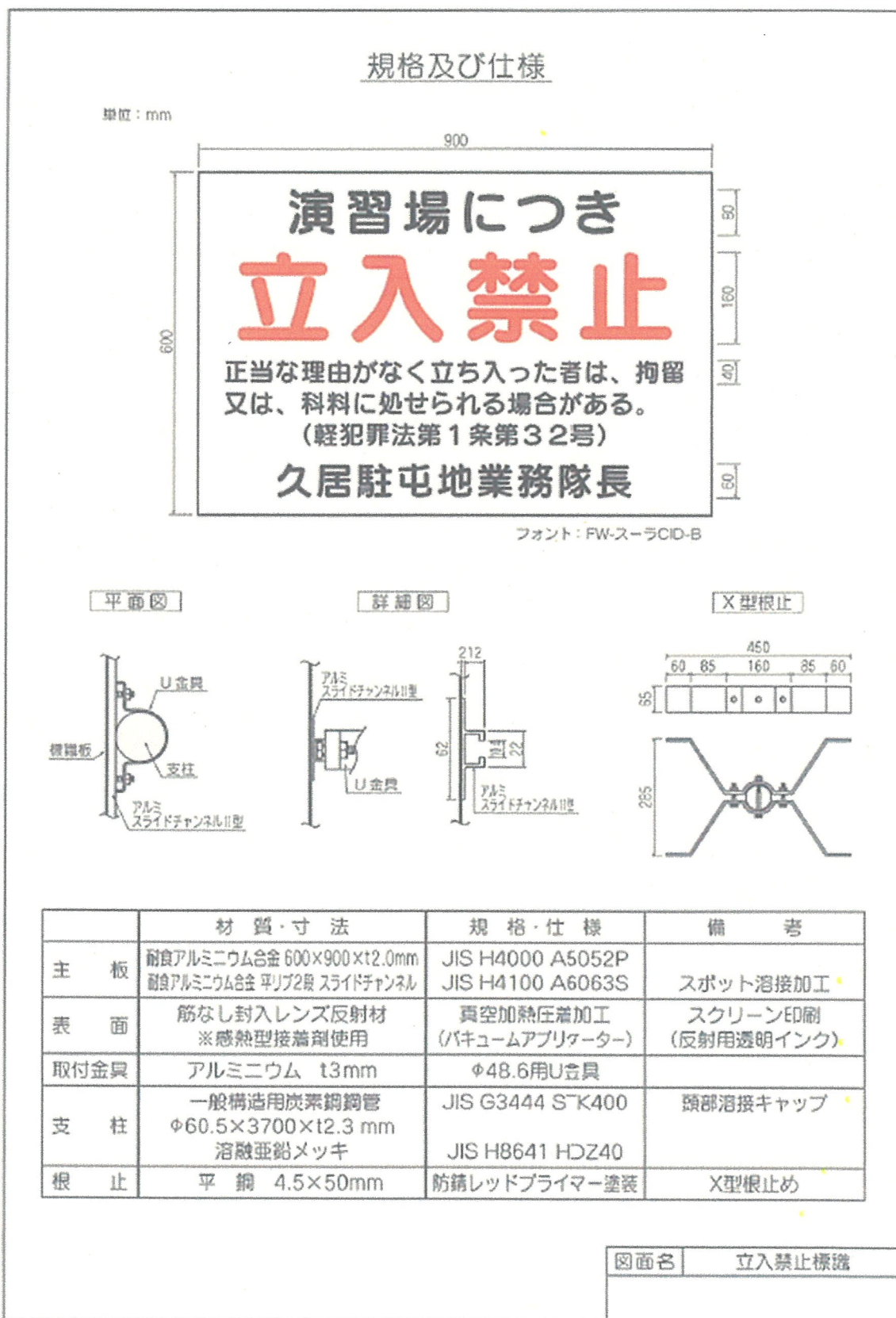
付図1-演習場立入禁止標識規格
