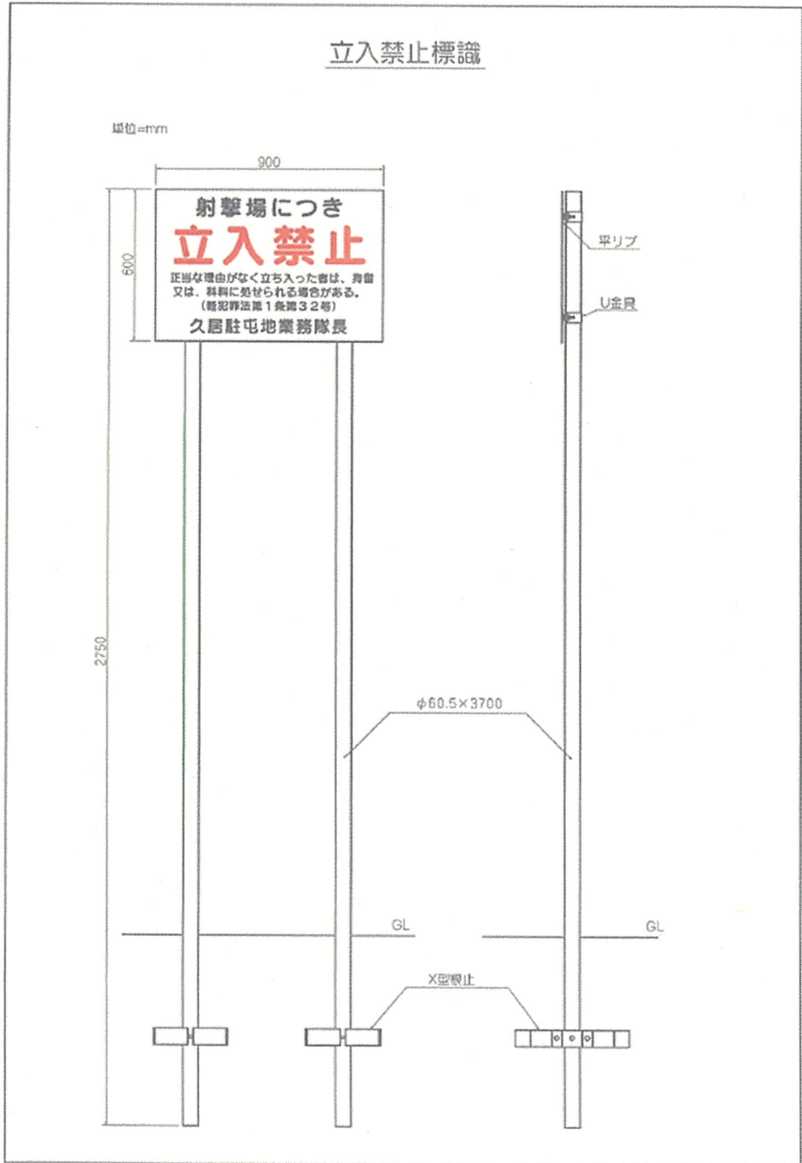
付図4-射撃場立入禁止標識外観、形状及び寸法
