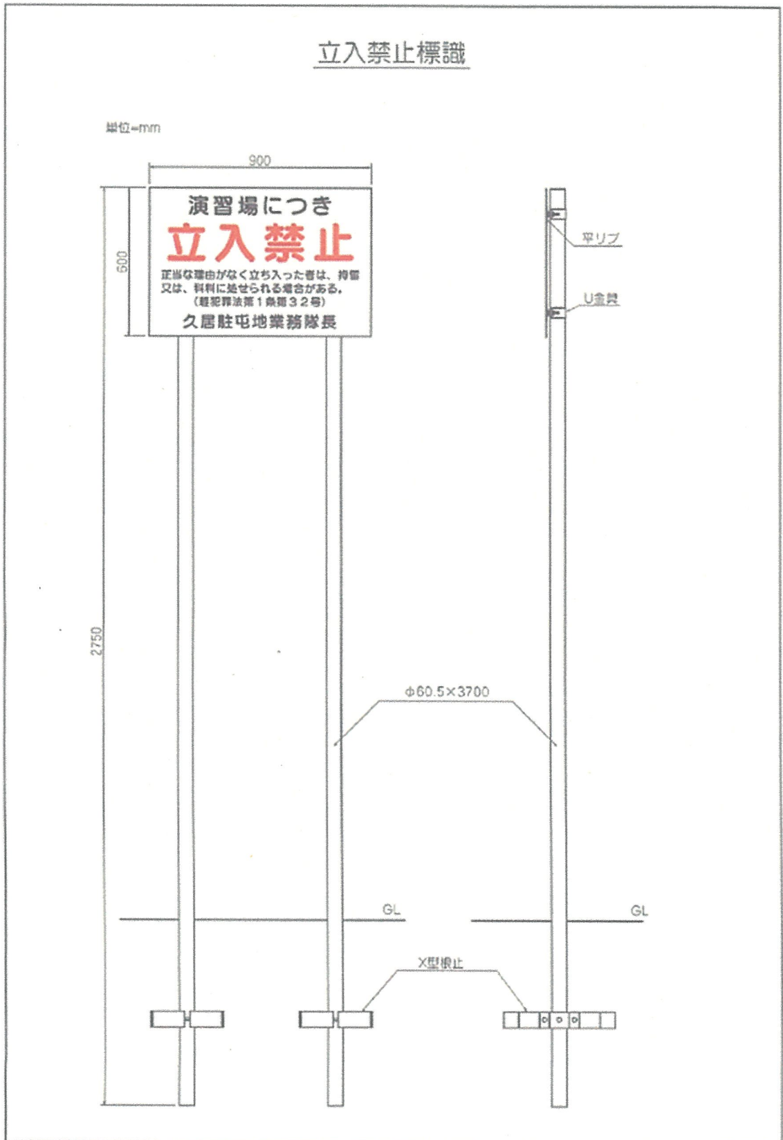
付図3-演習場立入禁止標識外観、形状及び寸法
