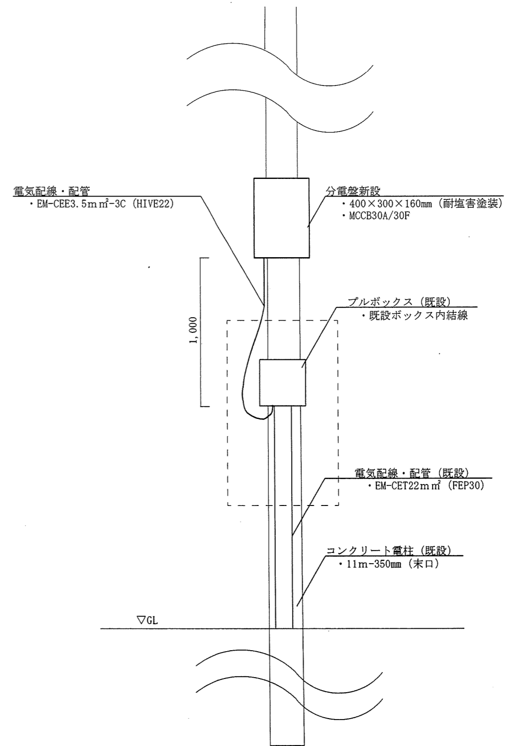
装柱B 詳細図
