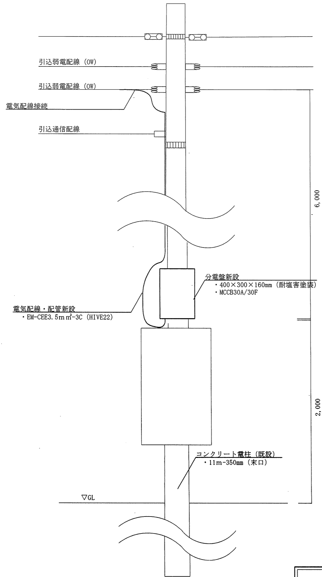
装柱A 詳細図
