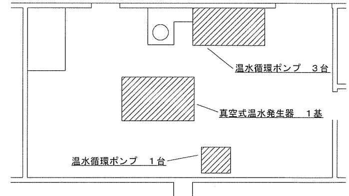
277号建物機械室平面図 1/X
