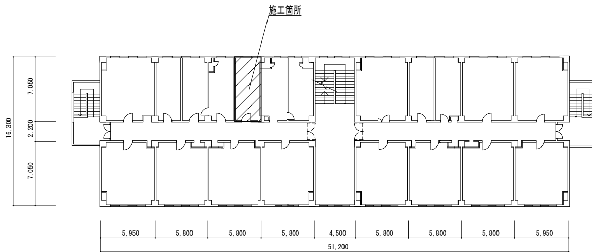
1号1階平面図 S=1/300
