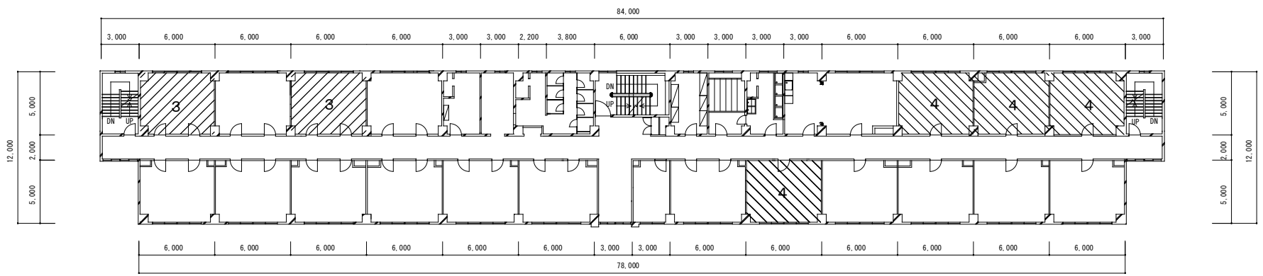
117号4階平面図
