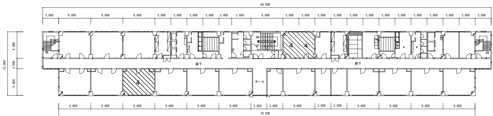
117号5階平面図
