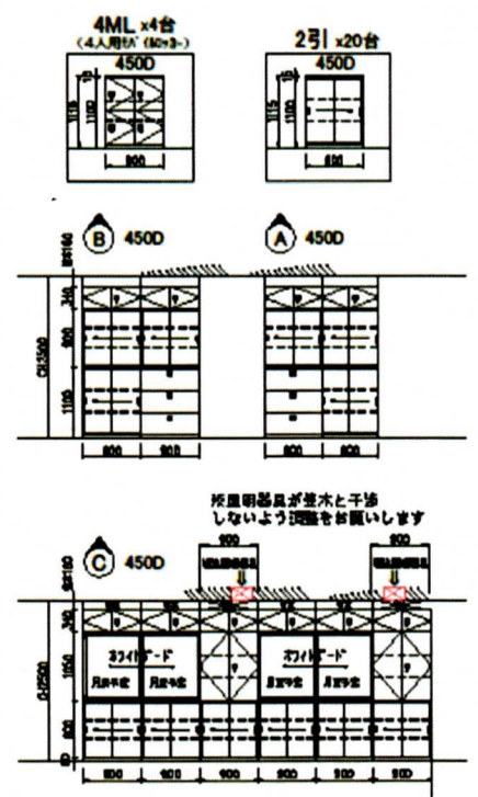
◆収納展開図 (S=1/80)
