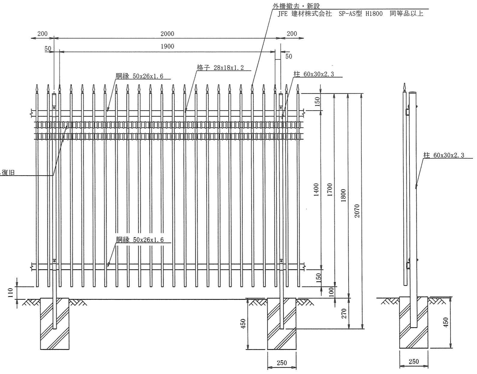
外柵立面図 S=1/20
