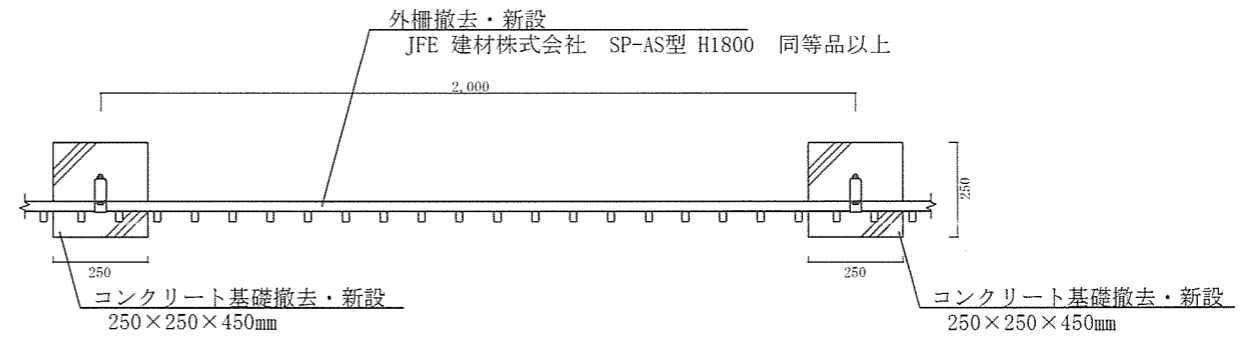
外柵平面図 S=1/20
