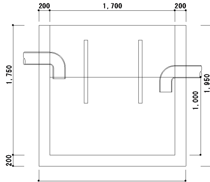
2,100 断面図
