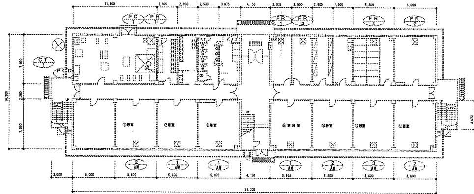
61号隊舎1階平面図 1/500
