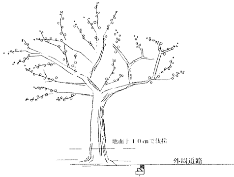
樹木伐採基準図 S=1:X
