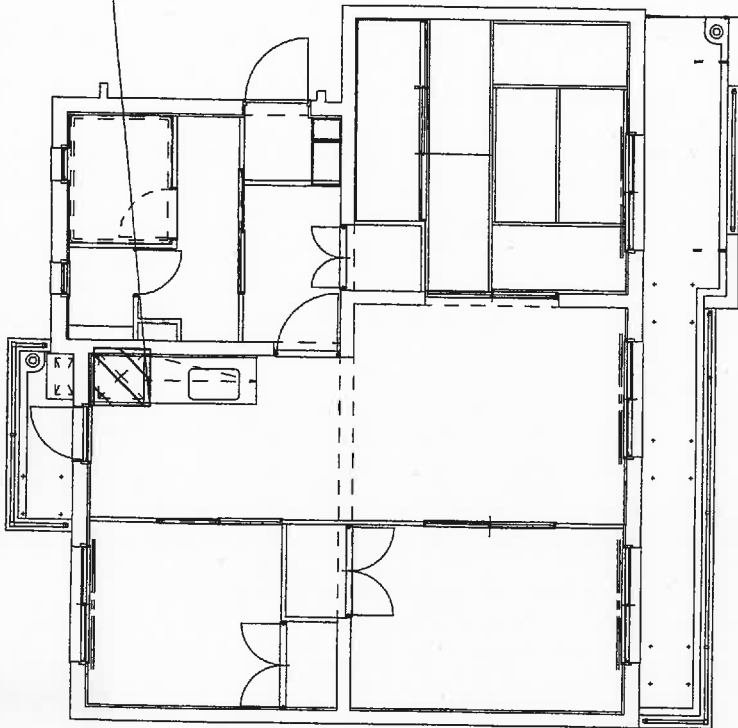
1～7号棟平面図
