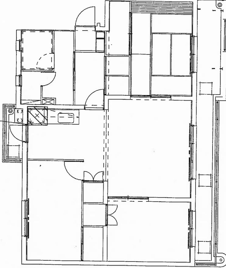
8号棟平面図
