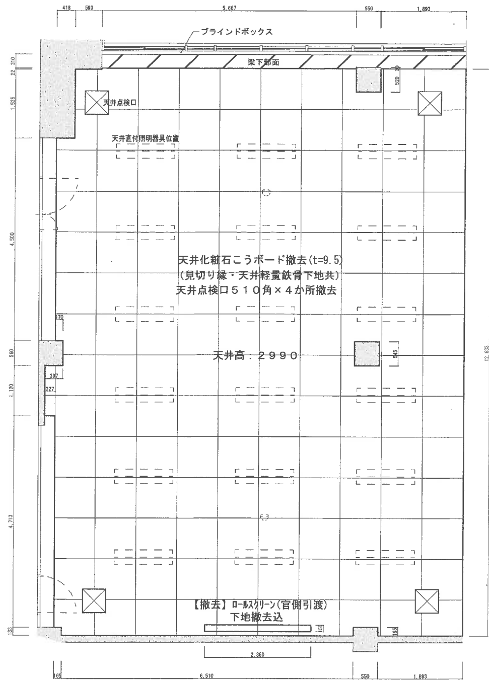
既設【撤去】中教場天井伏せ図
