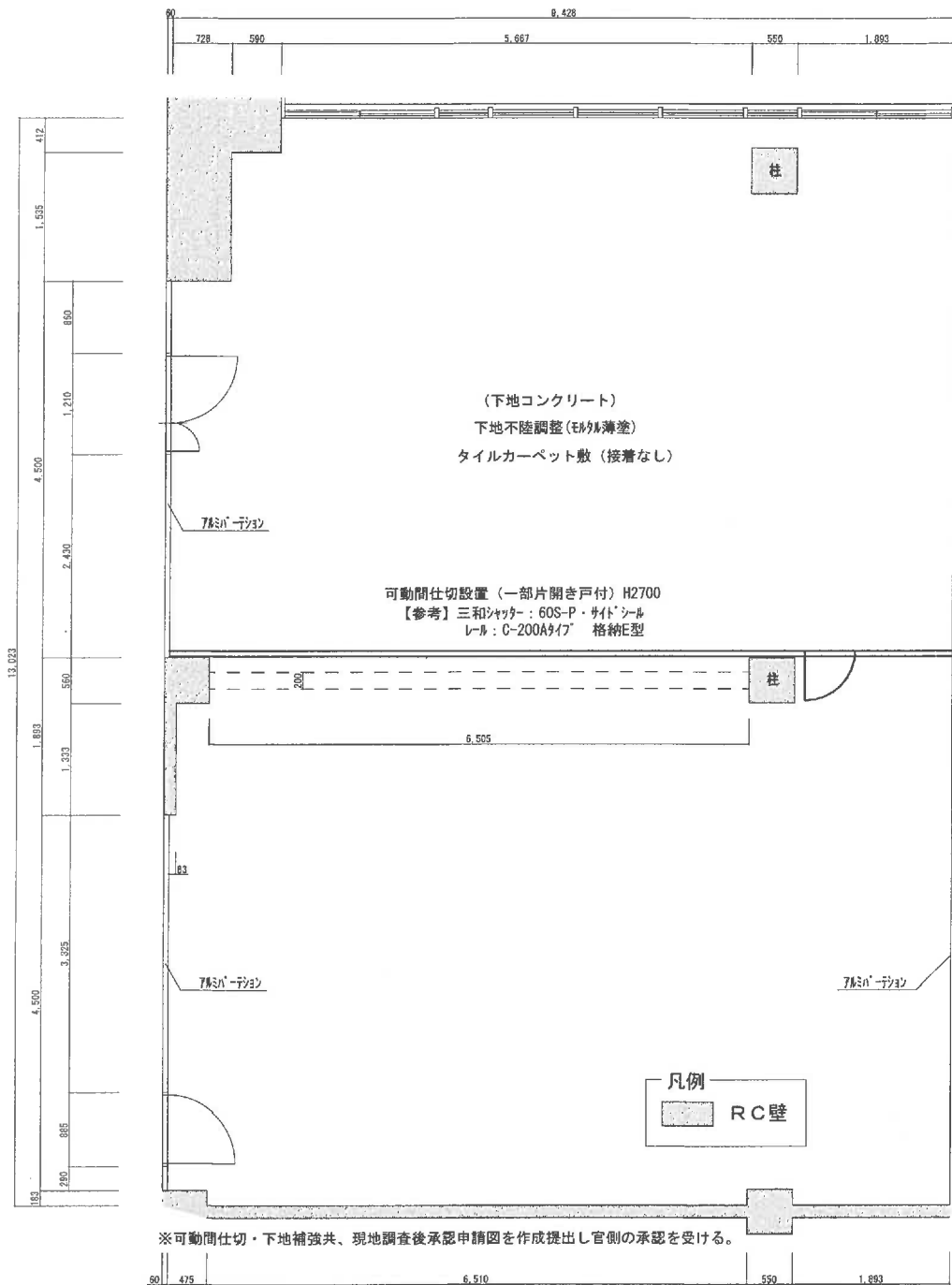
【改修】中教場平面図
