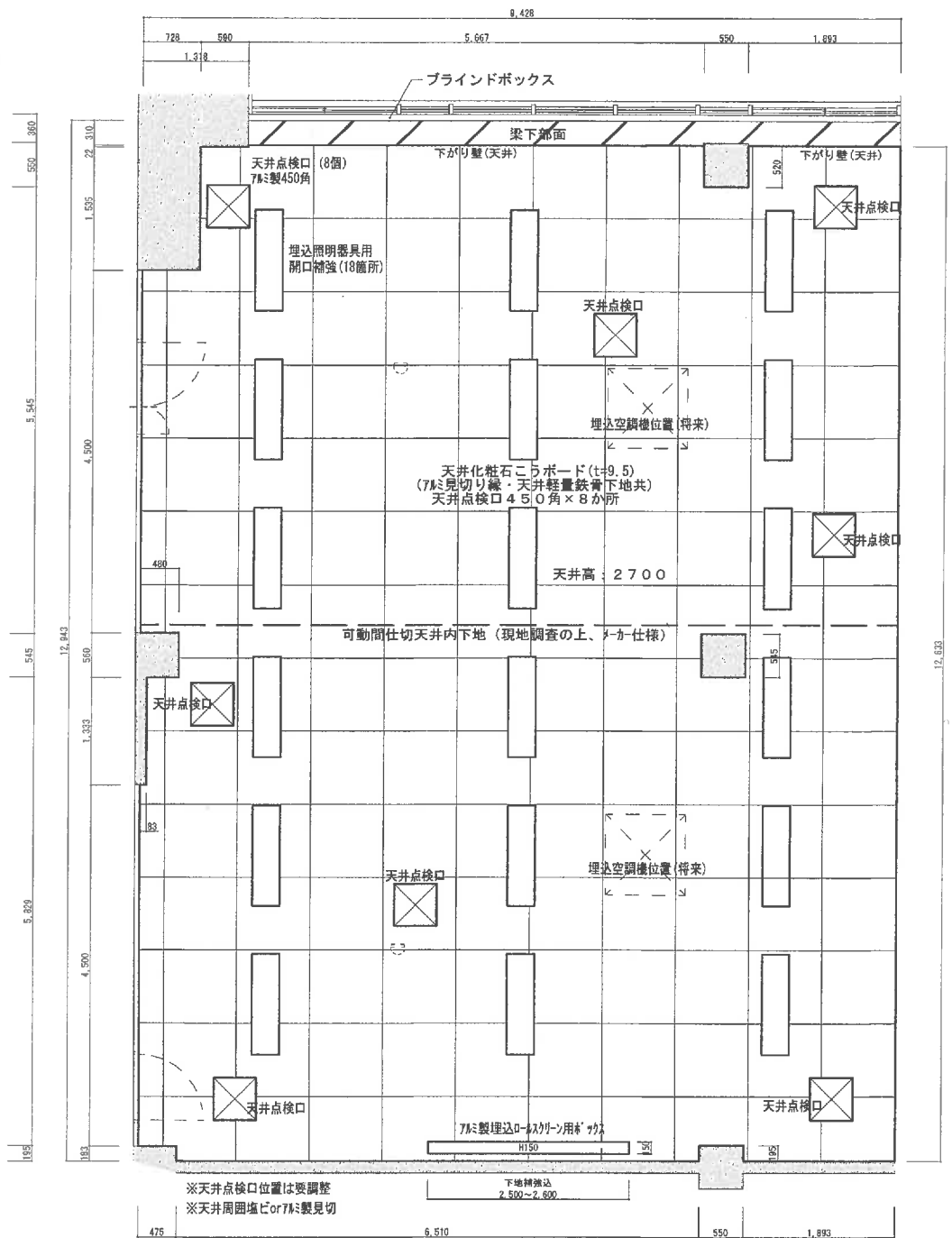
【改修】中教場天井伏せ図
