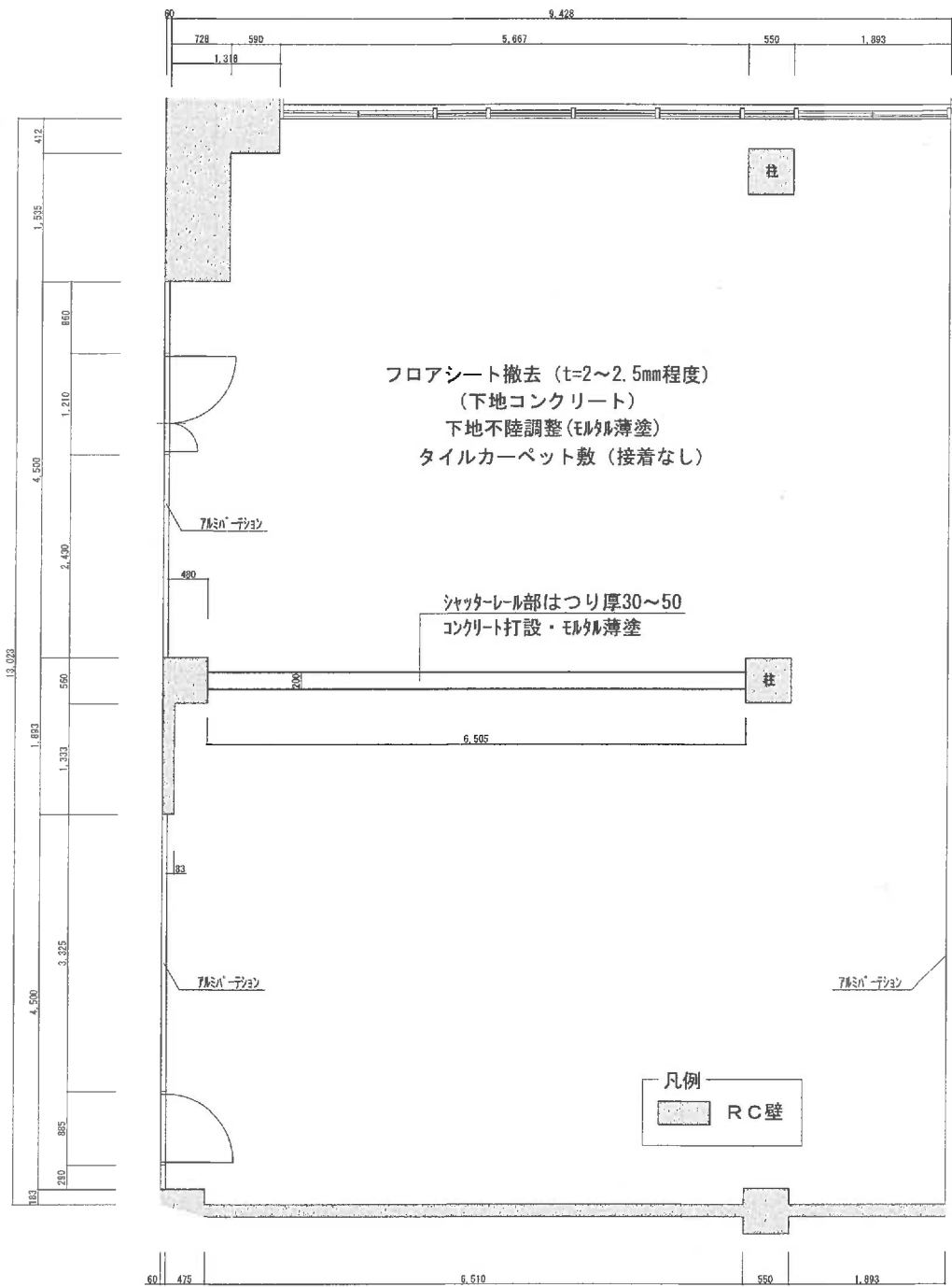
既設【撤去】中教場平面図
