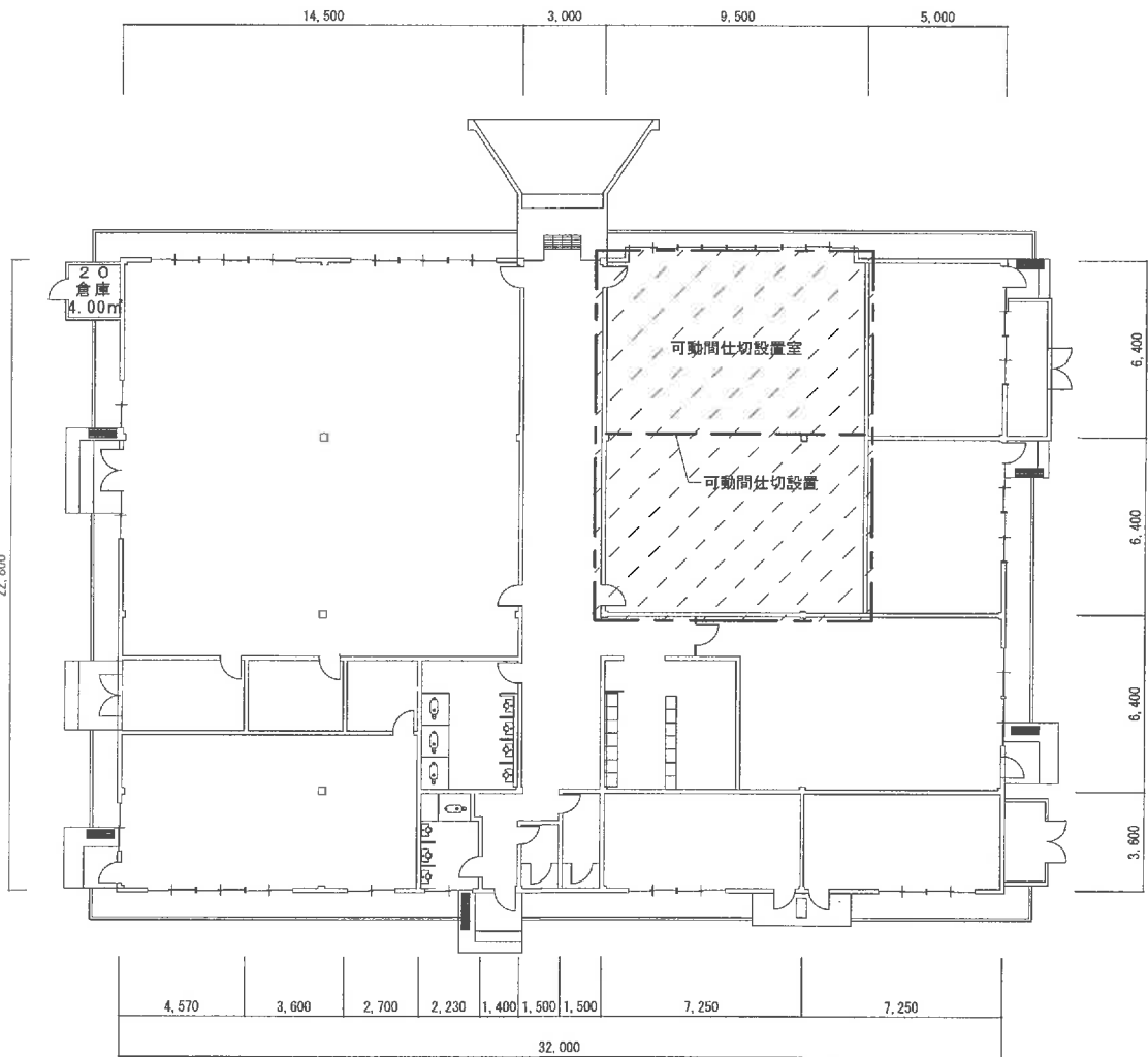
31号建物平面図 S=1:200
