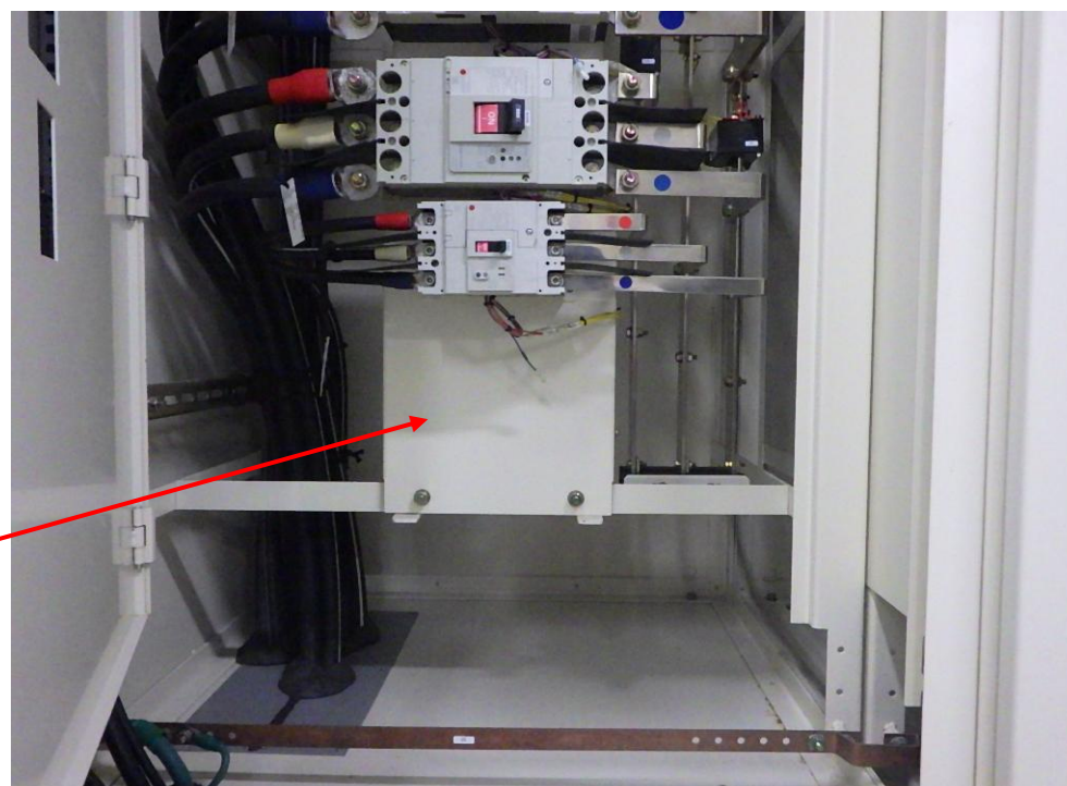
配線用遮断器新設個所拡大写真
