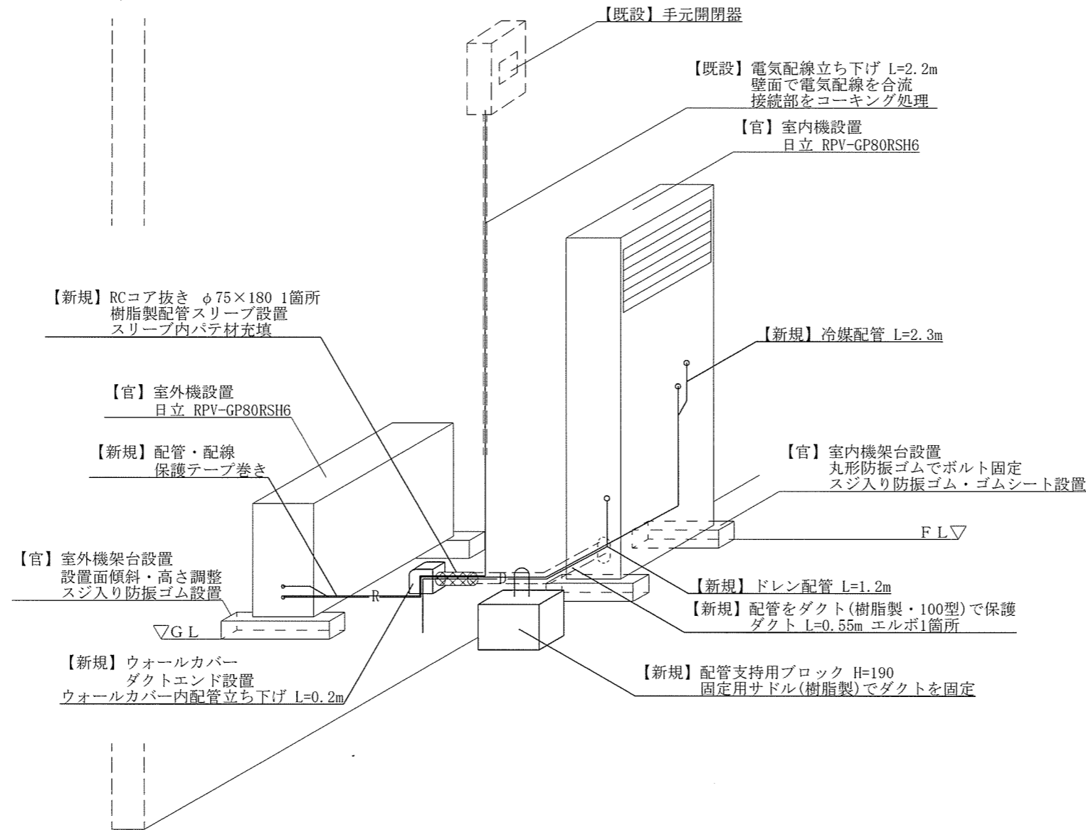
機器設置詳細図
