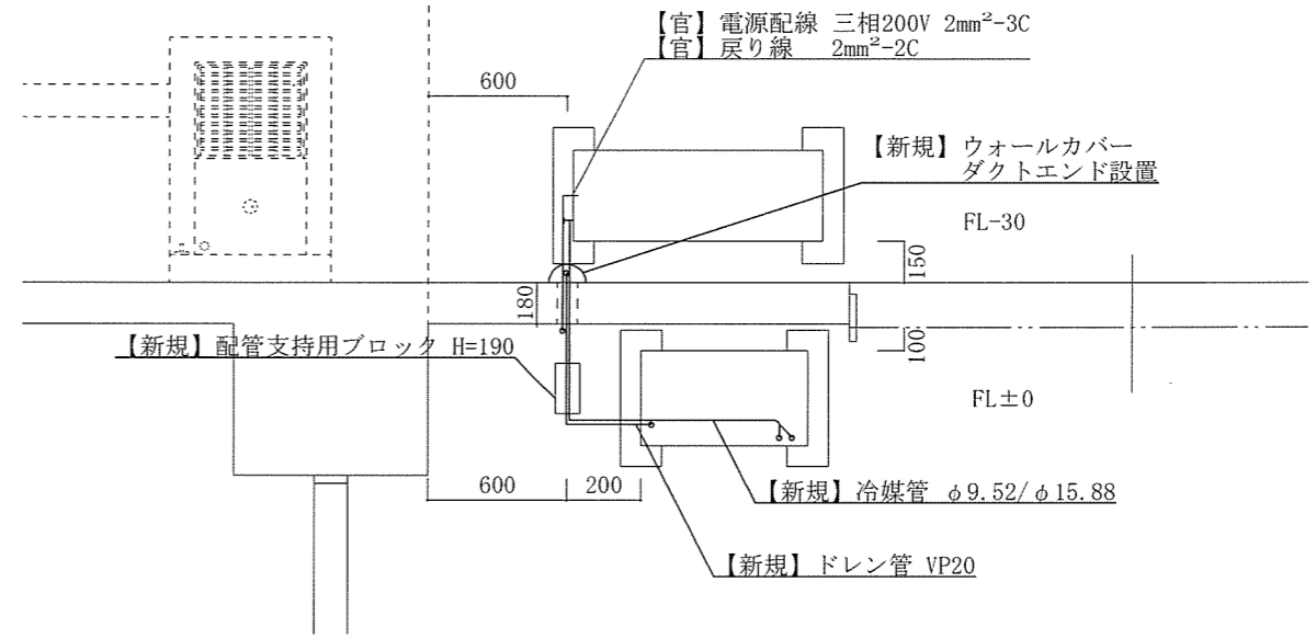
詳細図
