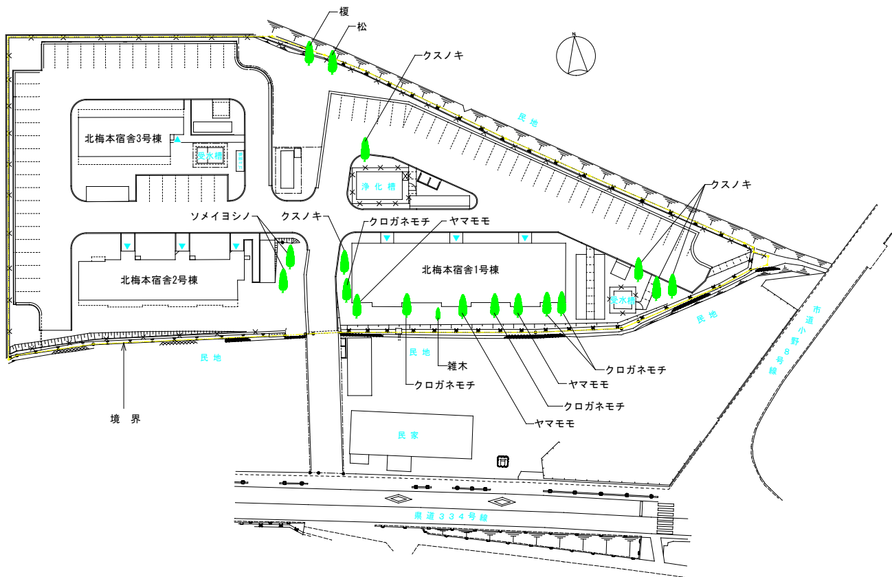
北梅本宿舎配置図 S=1/100
