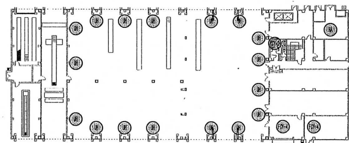
1階平面図 S=1/600
