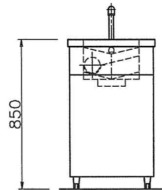
左側面図
