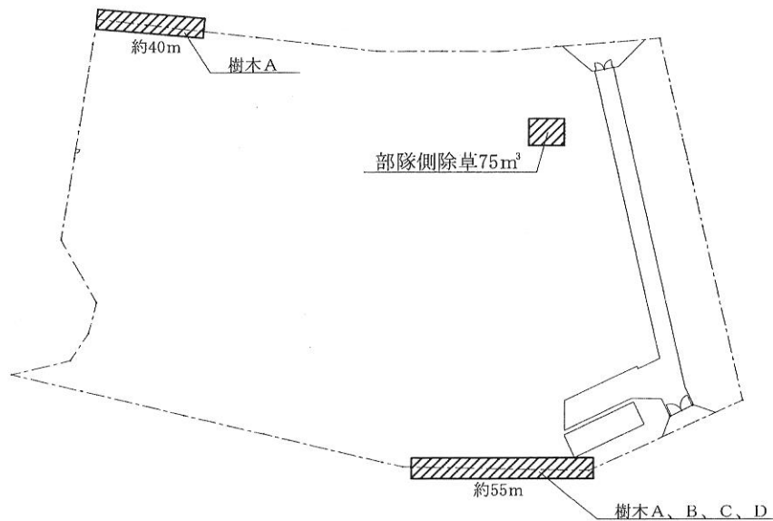
小幡訓練場配置図 S=1/2500
