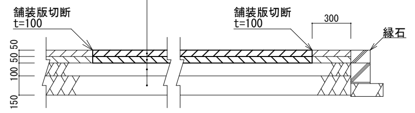
A-A' 舗装断面図 (基準) S=1:30
