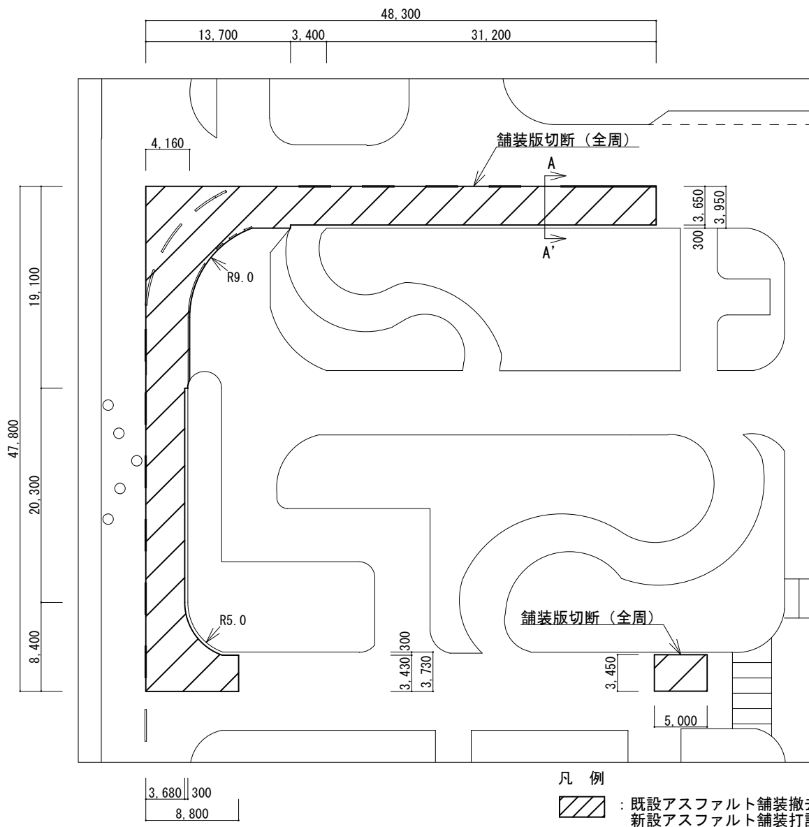
アスファルト舗装補修 平面図 S=1:500
