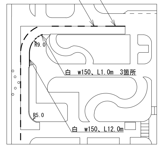
区画線塗装 平面図 S=1:1000
