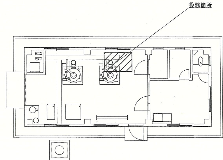
28号生活隊舎2階平面図 S=1:400
