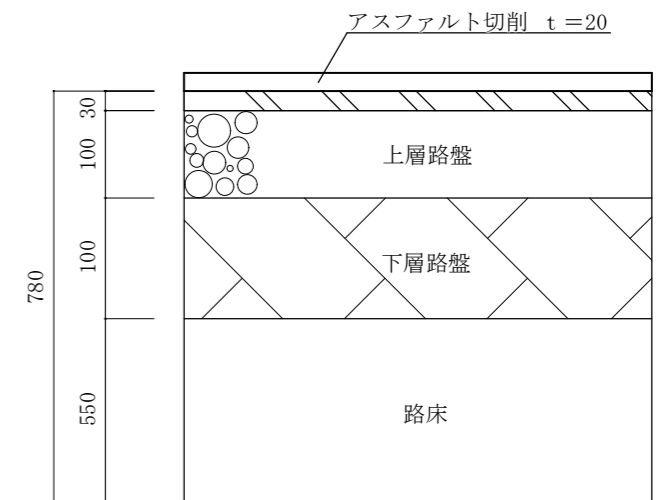
切削断面図 S=1/NS
