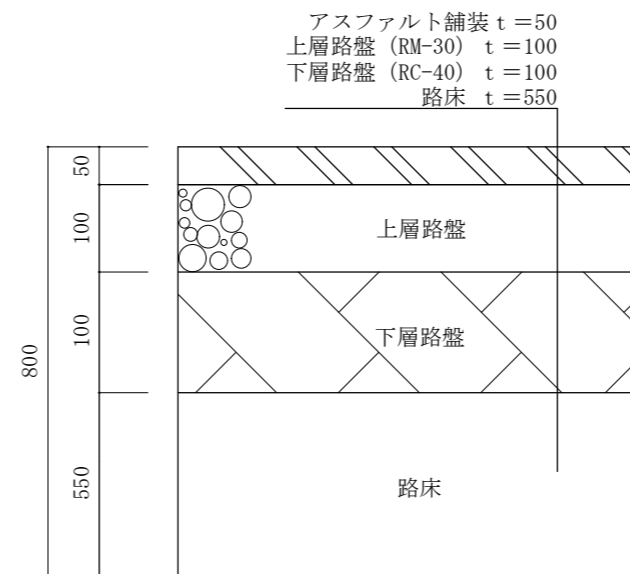
既設断面図 S=1/NS
