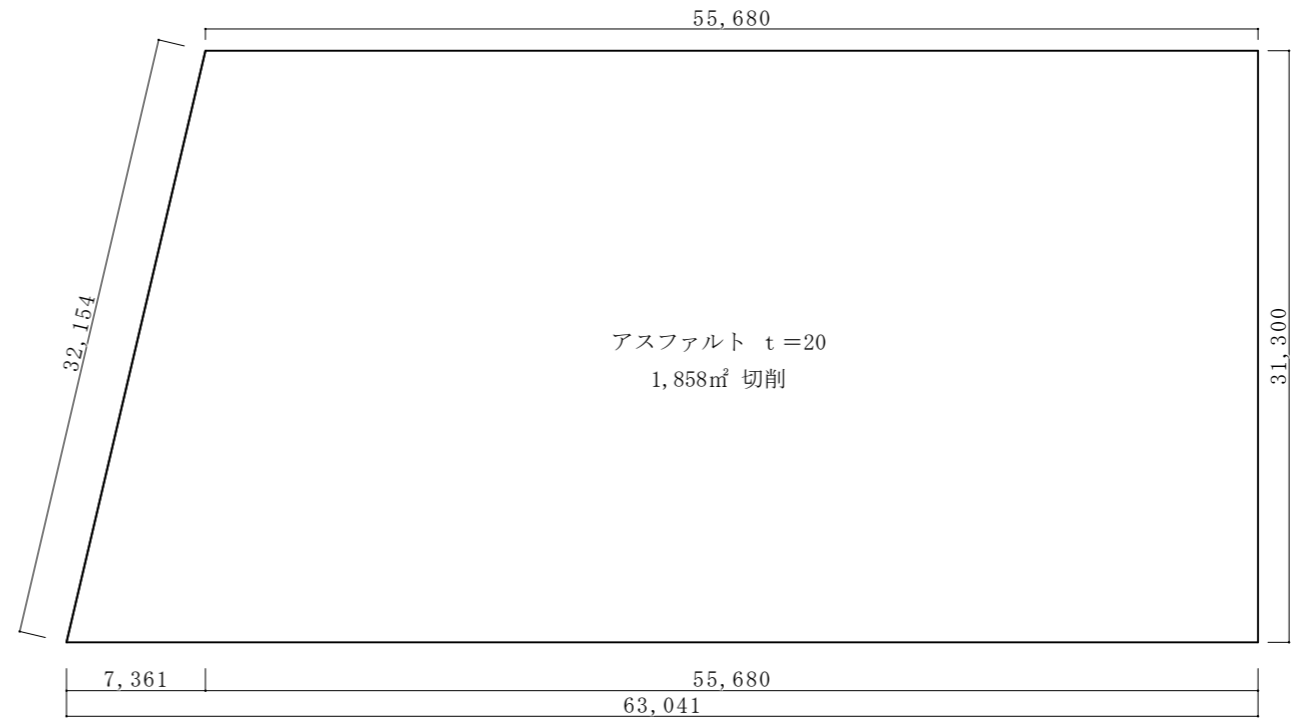
A s 切削平面図 S=1/400
