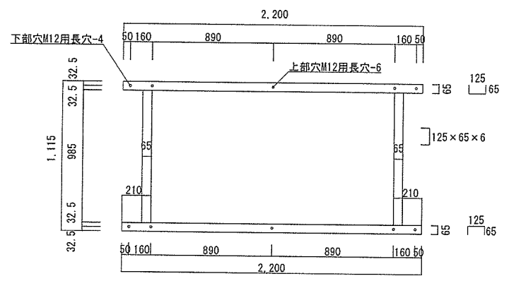
エコキュート架台詳細図 S=1/25
