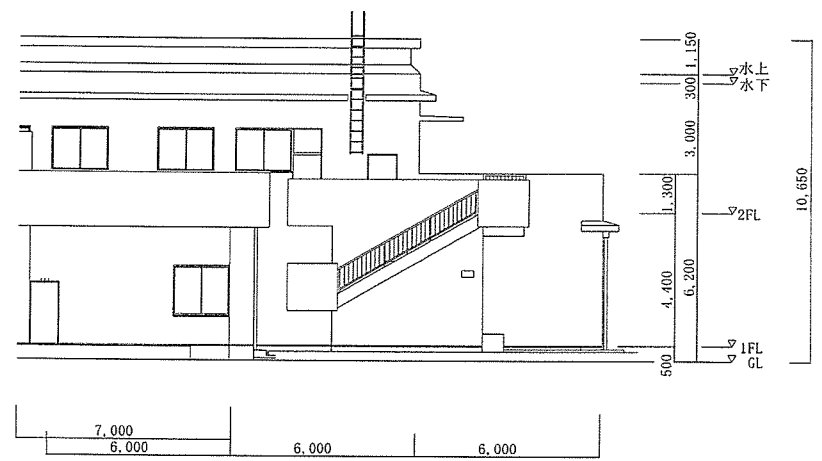
2号北側立面図 S=1/500
