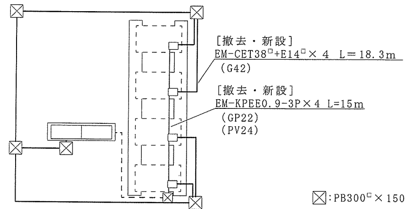
電源・通信配線詳細図
