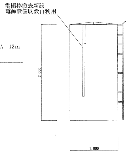
A~A' 断面図 1/40
