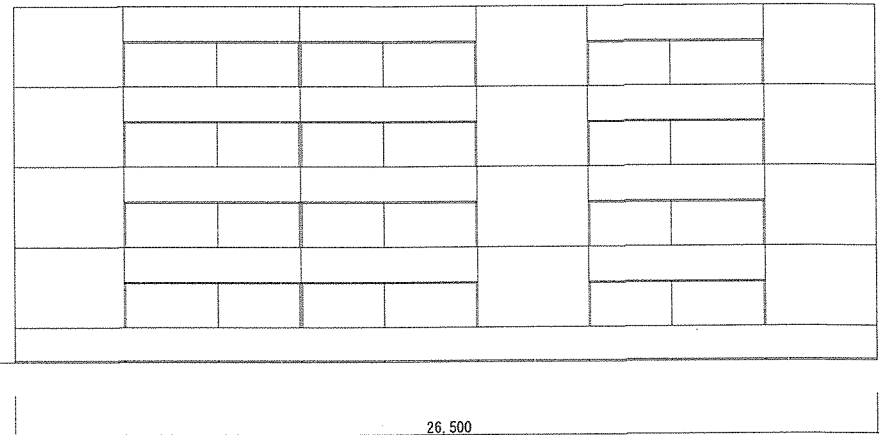
公務員宿舎断面図 1 / 2 5 0
