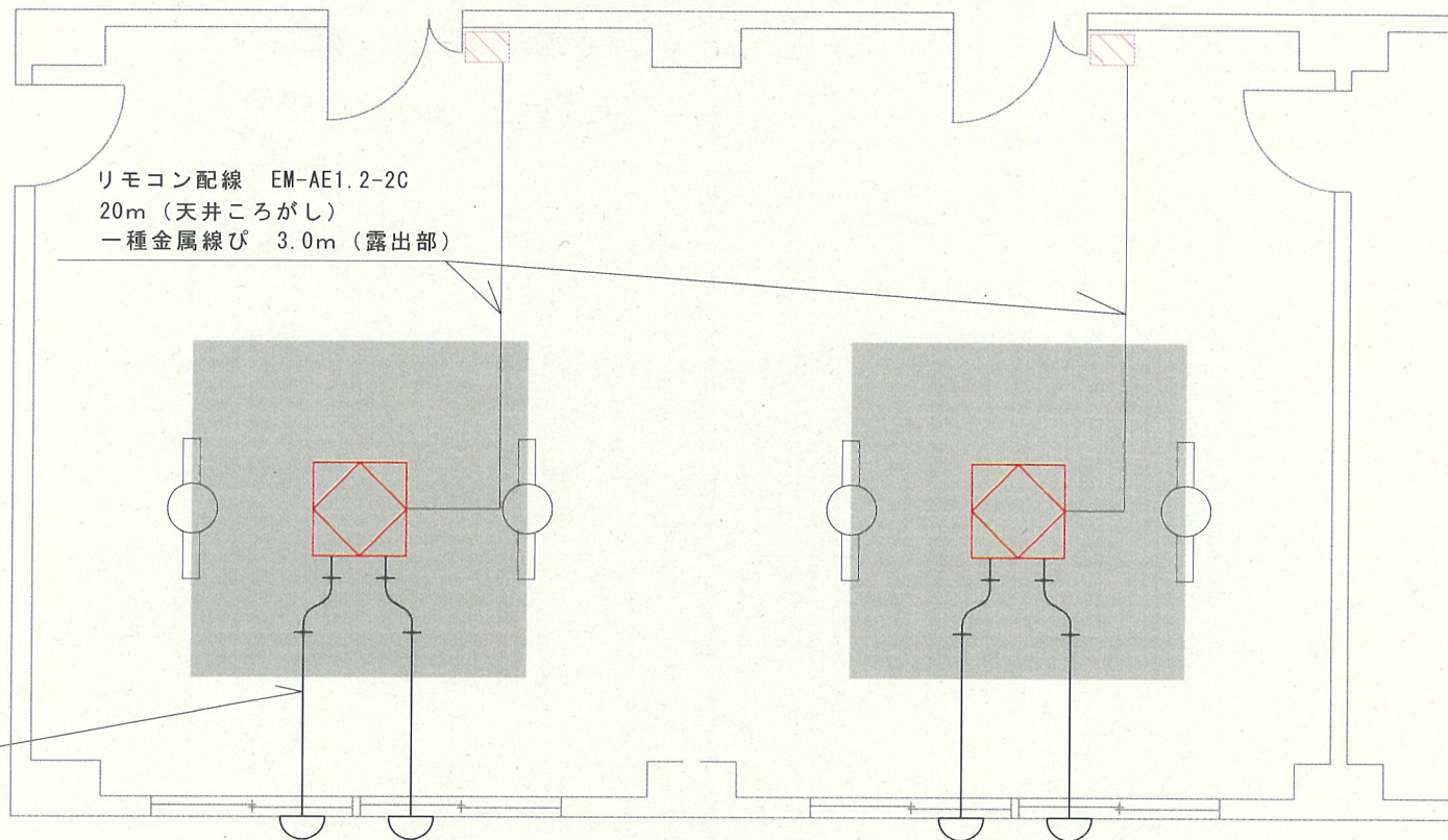
換気設備詳細図 S=1/50
