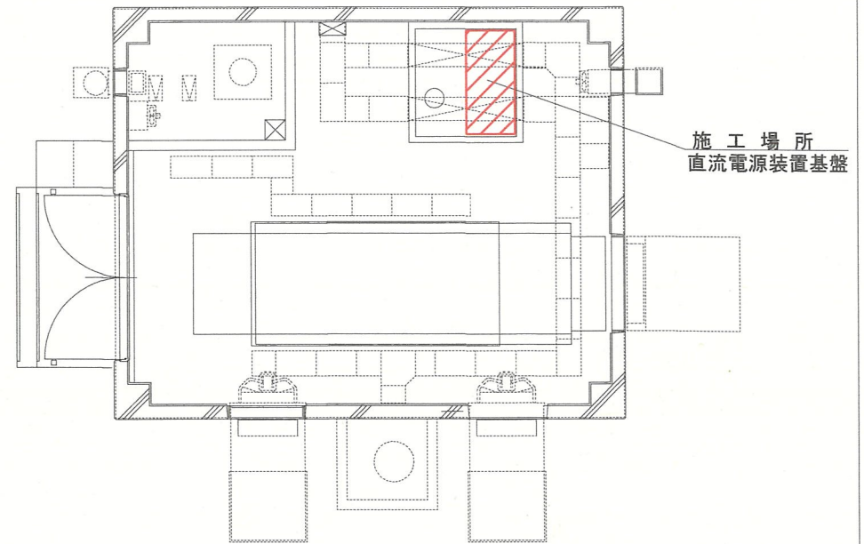
施工場所詳細図 S=1:100
