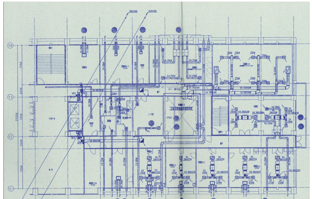
ダクト系統図
