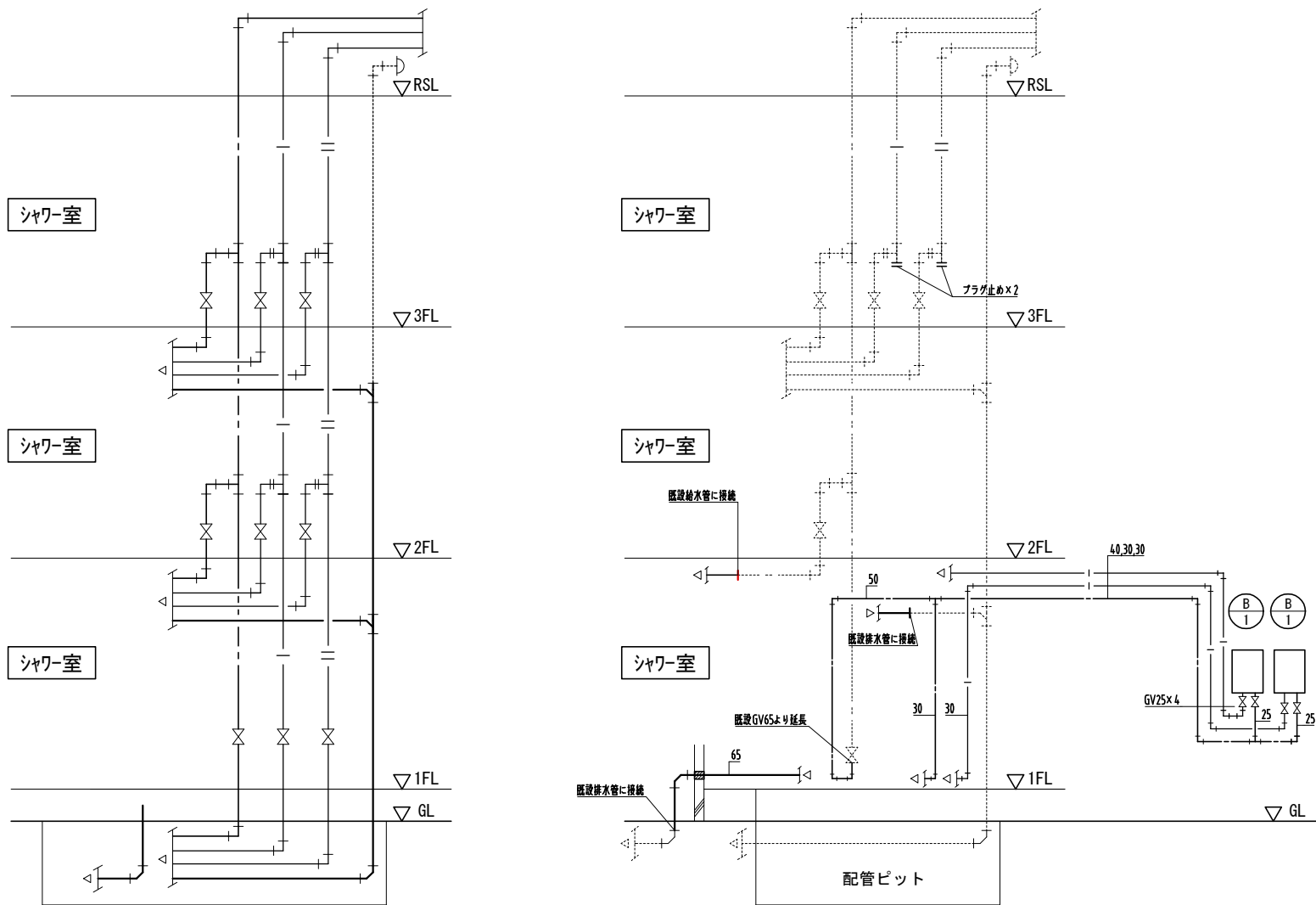
系統図（現況撤去）給排水設備 1:50
