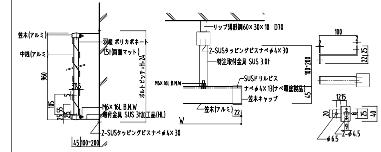
断面図 1:20
