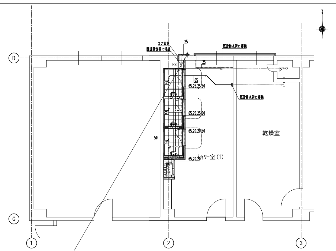
2階平面詳細図 (改修) 給排水設備 1:50
