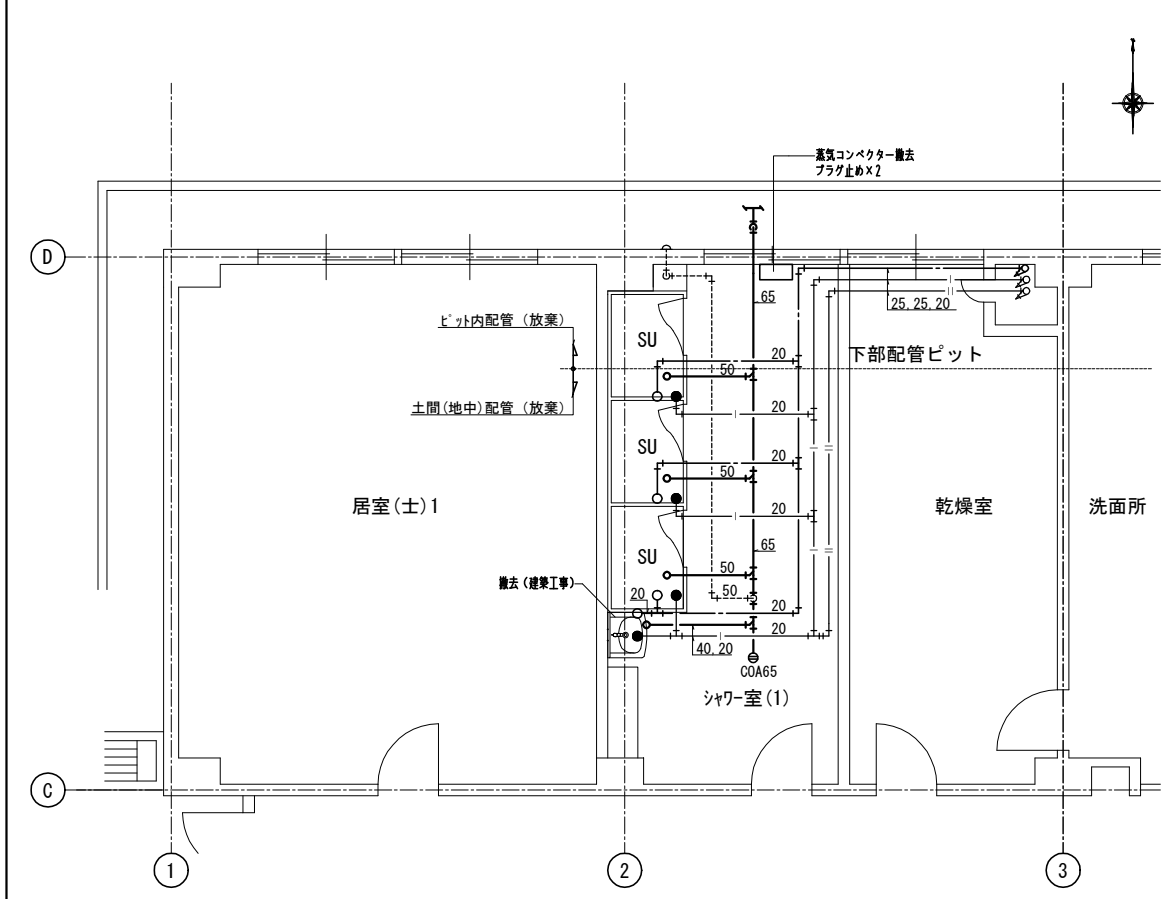
1階平面詳細図 (現況・撤去) 給排水設備 1:50
