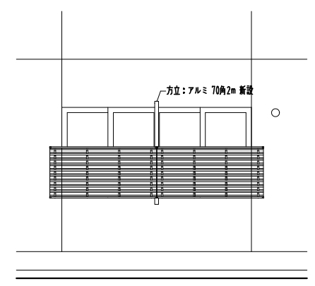
部分立面図 (改修) 1:50
