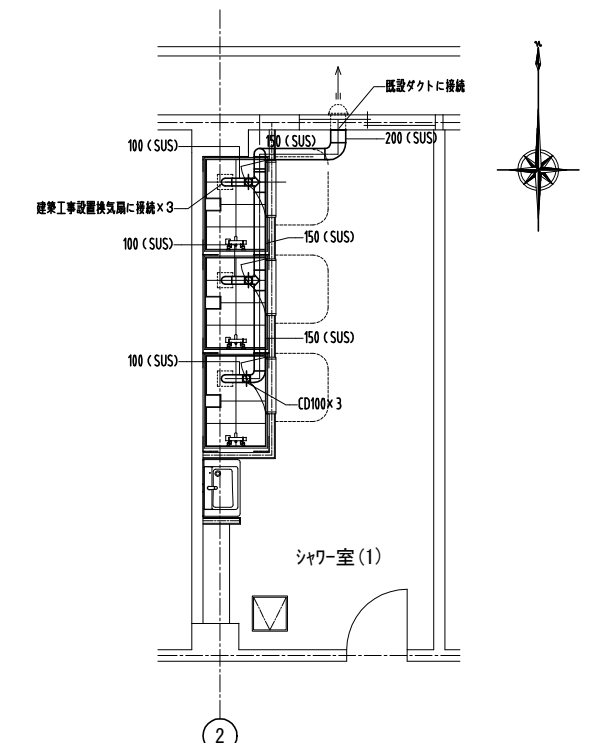
2階平面詳細図（改修）換気設備 1:50
