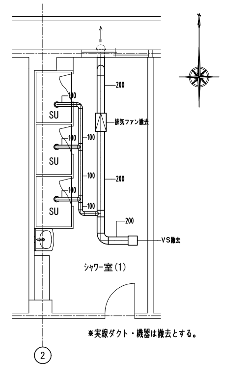
2階平面詳細図（現況・撤去）換気設備 1:50
