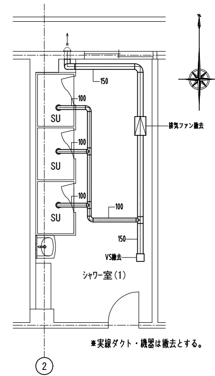
1階平面詳細図（現況・撤去）換気設備 1:50
