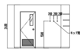
1・2階C面展開図 (改修) 1:50
