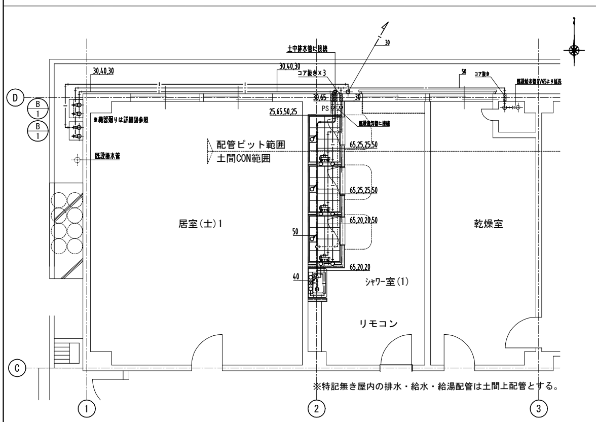
1階平面詳細図 (改修) 給排水設備 1:50
