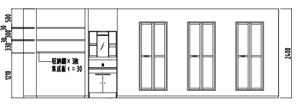
1・2階D面展開図 (改修) 1:50
