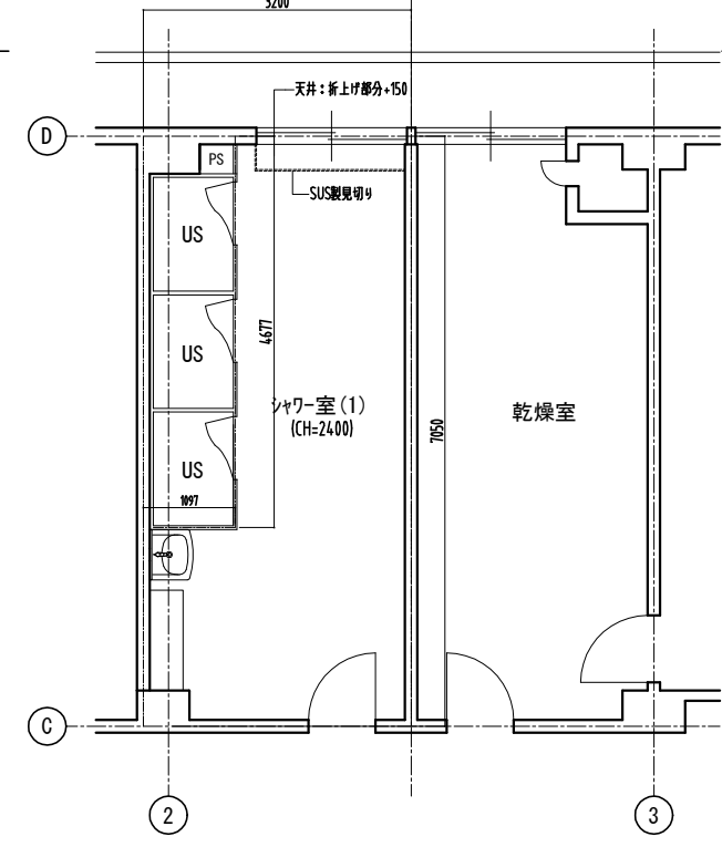
2階平面詳細図 (現況・撤去) 1:50
