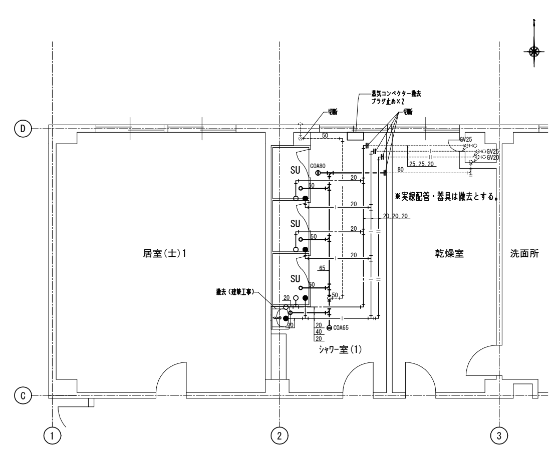
2階平面詳細図 (現況・撤去) 給排水設備 1:50
