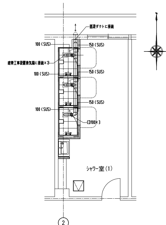
1階平面詳細図（改修）換気設備 1:50
