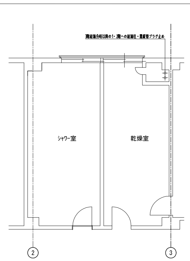
3階平面詳細図 (改修) 給排水設備 1:50
