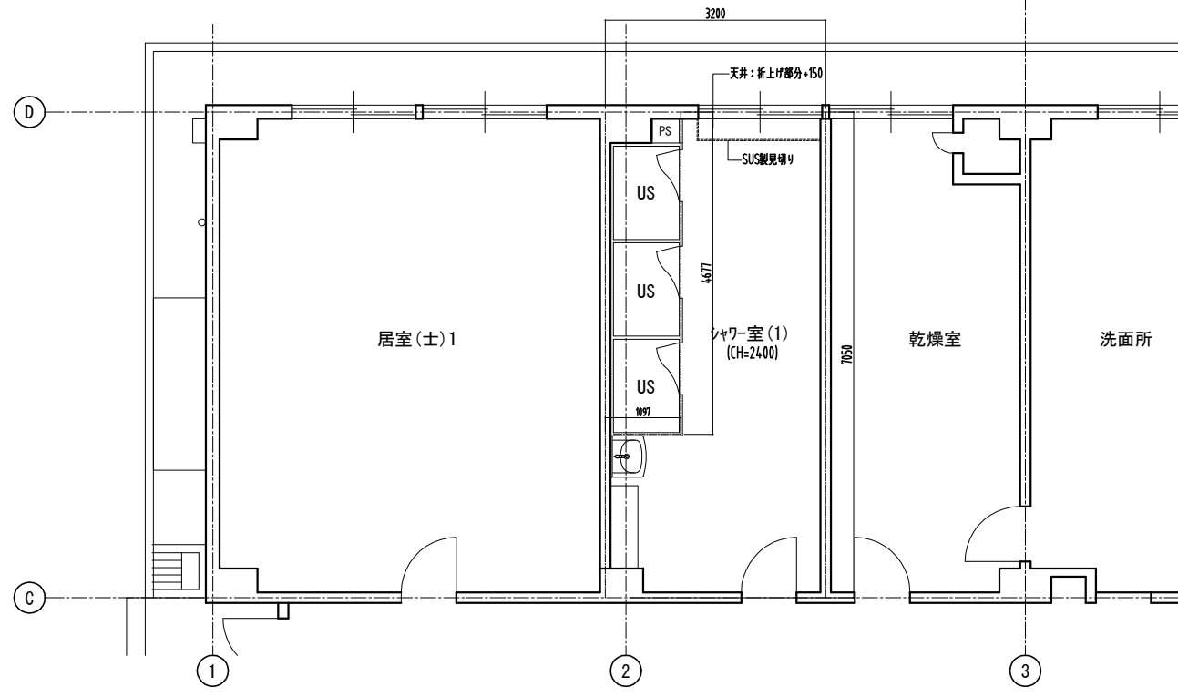
1階平面詳細図 (現況・撤去) 1:50
