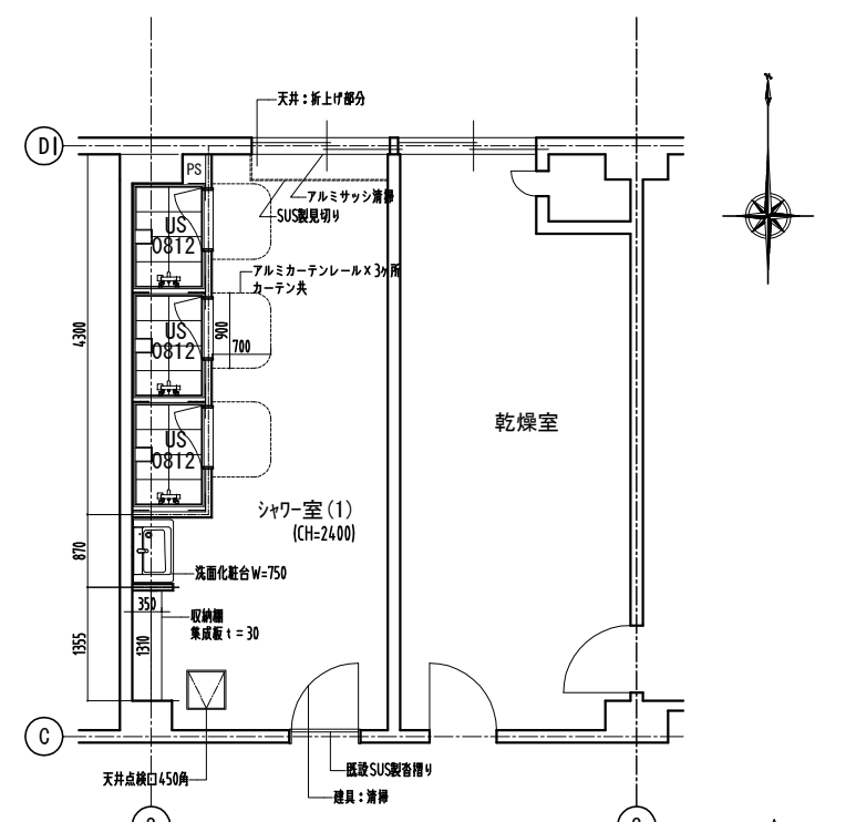
2階平面詳細図 (改修) 1:50
