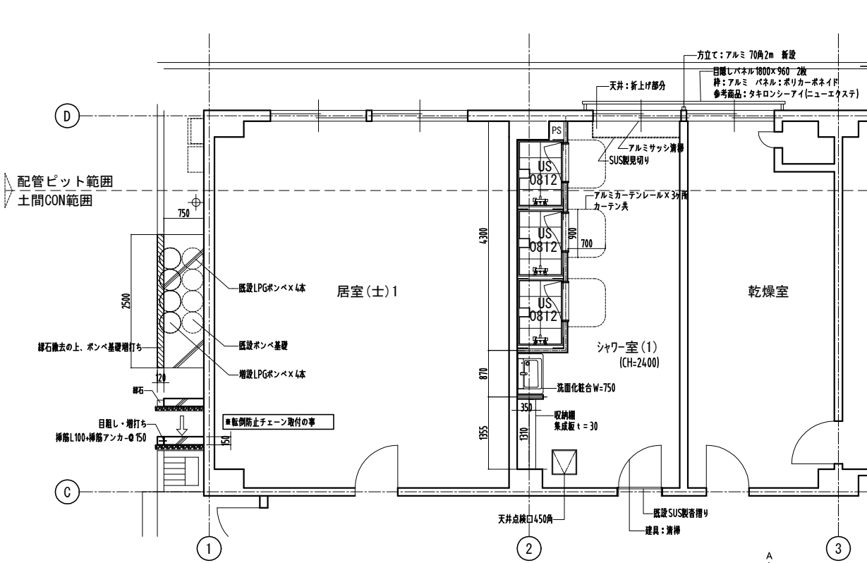
1階平面詳細図 (改修) 1:50
