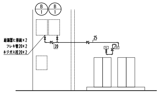
部分詳細図（改修）ガス設備 1:50
