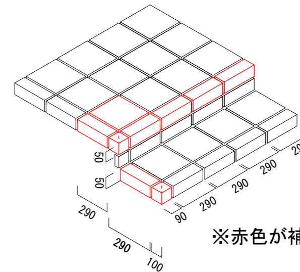
タイル補修詳細図 1 : 1 0
