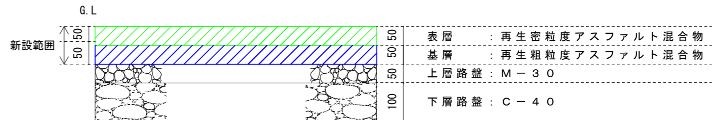
補修後 舗装断面図 1 : 10
