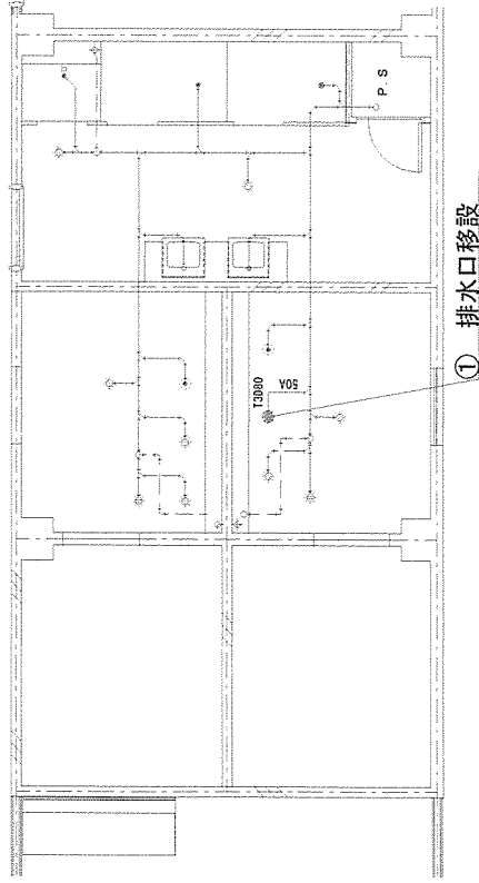
改修前 排水図 1/100
