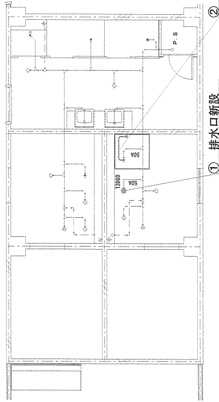
改修後 排水図 1/100
