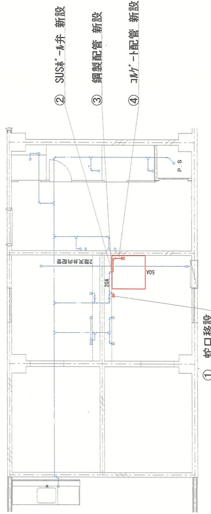
改修後 給水図 1/100
