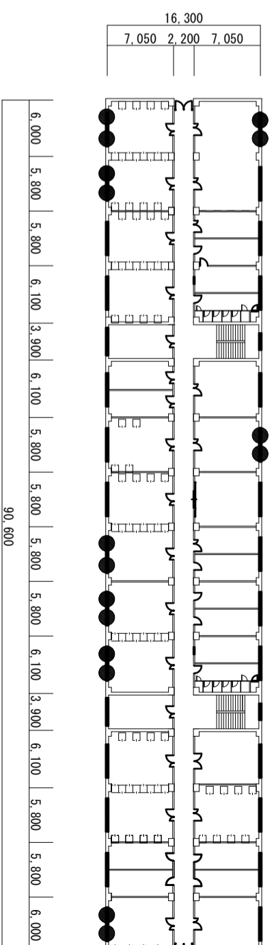
203号建物 3階平面図
