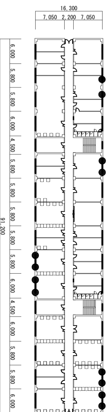
203号建物 4階平面図
