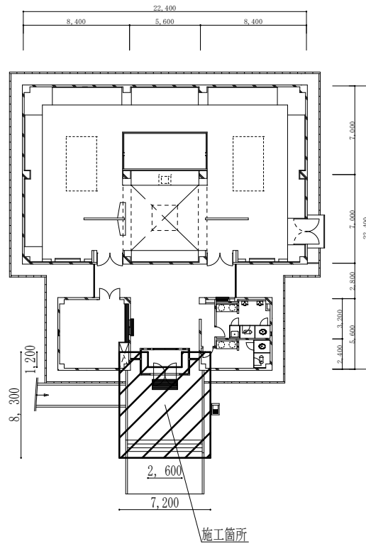
223号 平面図 S=1/300
