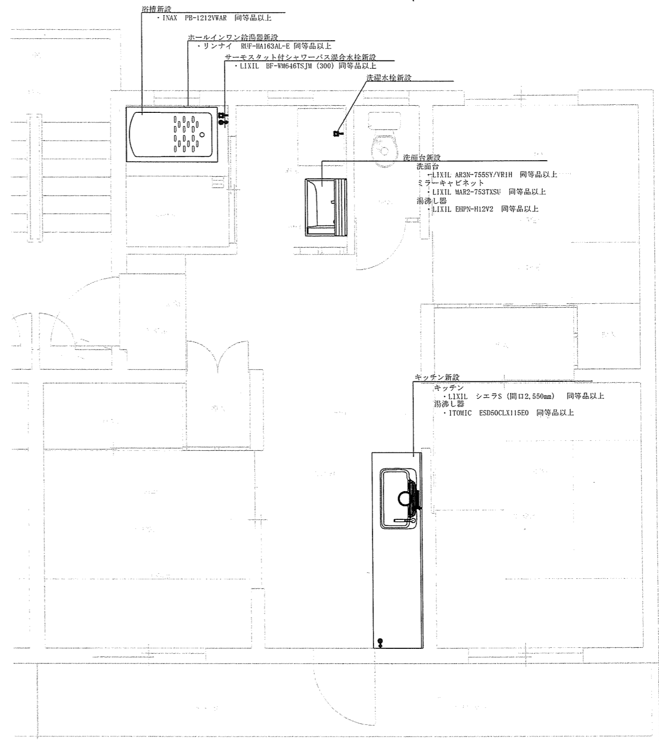
改修後平面図
