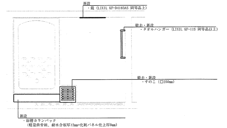
浴室改修前・後平面図 (付帯設備) S=1/30
