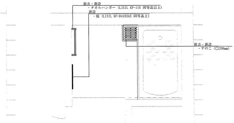
浴室改修前・後平面図 (付帯設備) S=1/30
