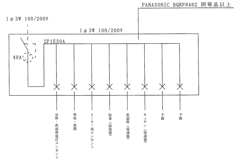
分電盤詳細図 (新設) S=1/X
