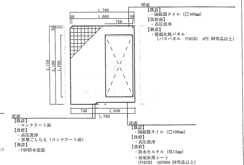
D面立面図 S=1/60
