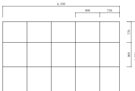
畳 (取替後) 平面図 S=1:50
