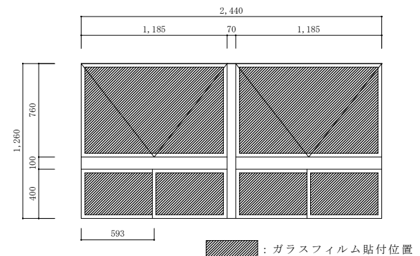
窓立面図 S=1:30
