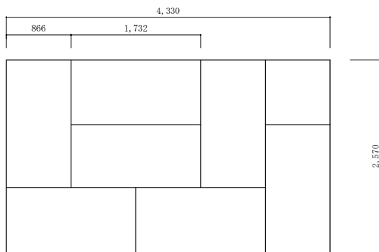
畳 (取替前) 平面図 S=1:50
