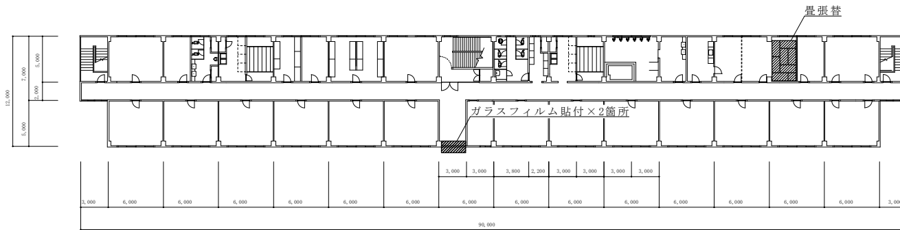
255号建物1階平面図 S=1:400
